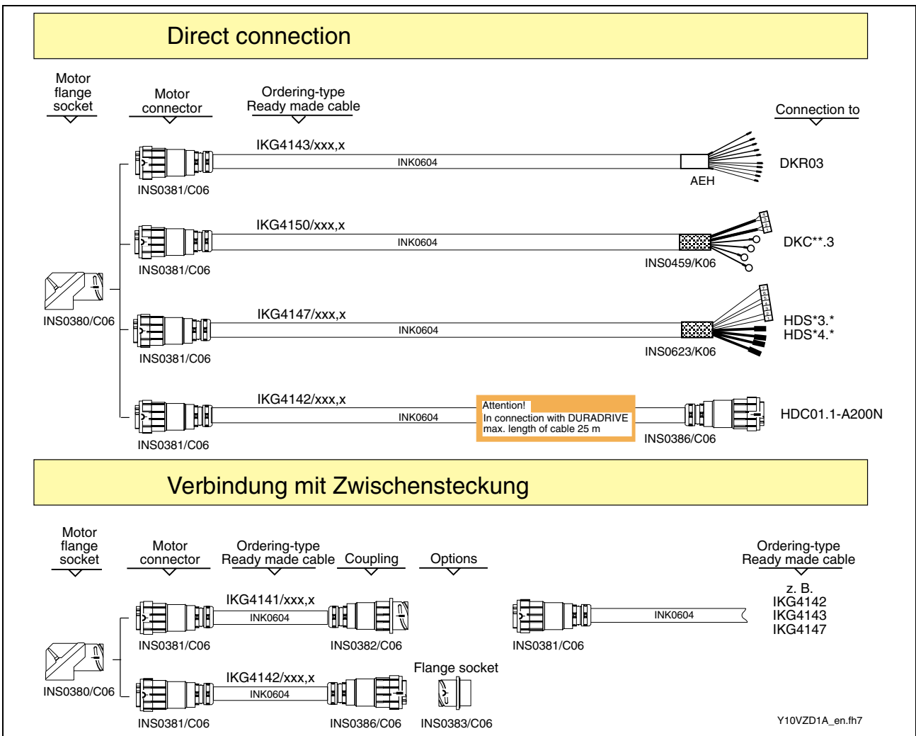
Fig. 17-9: Kabelauswahl INS0380 – 6,0mm 2
