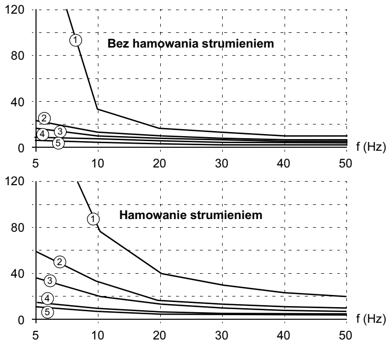
Rysunek 6-15 Moment hamujący silnika w procentach znamionowego momentu obrotowego w funkcji częstotliwości wyjściowej
