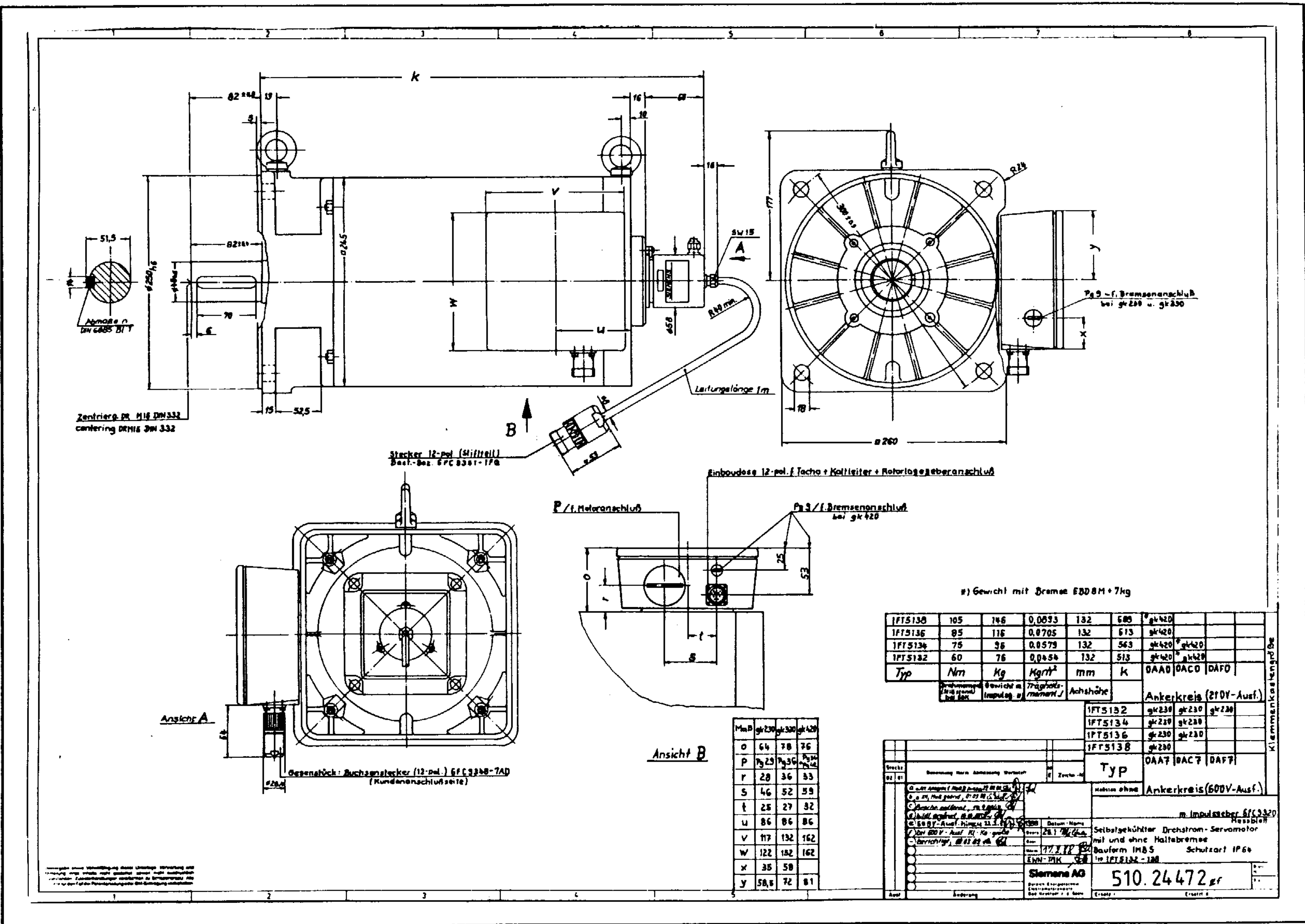
Bild 6.39 Maßblatt Drehstrom-Servomotoren 1FT5132 bis 1FT5138 mit Impulsgeber 6FC9320 - Bauforn IM B5 Bitte achten Sie auf die Zuordnung der Klemmenkastengrößen für die Ankerkreise 600V.
