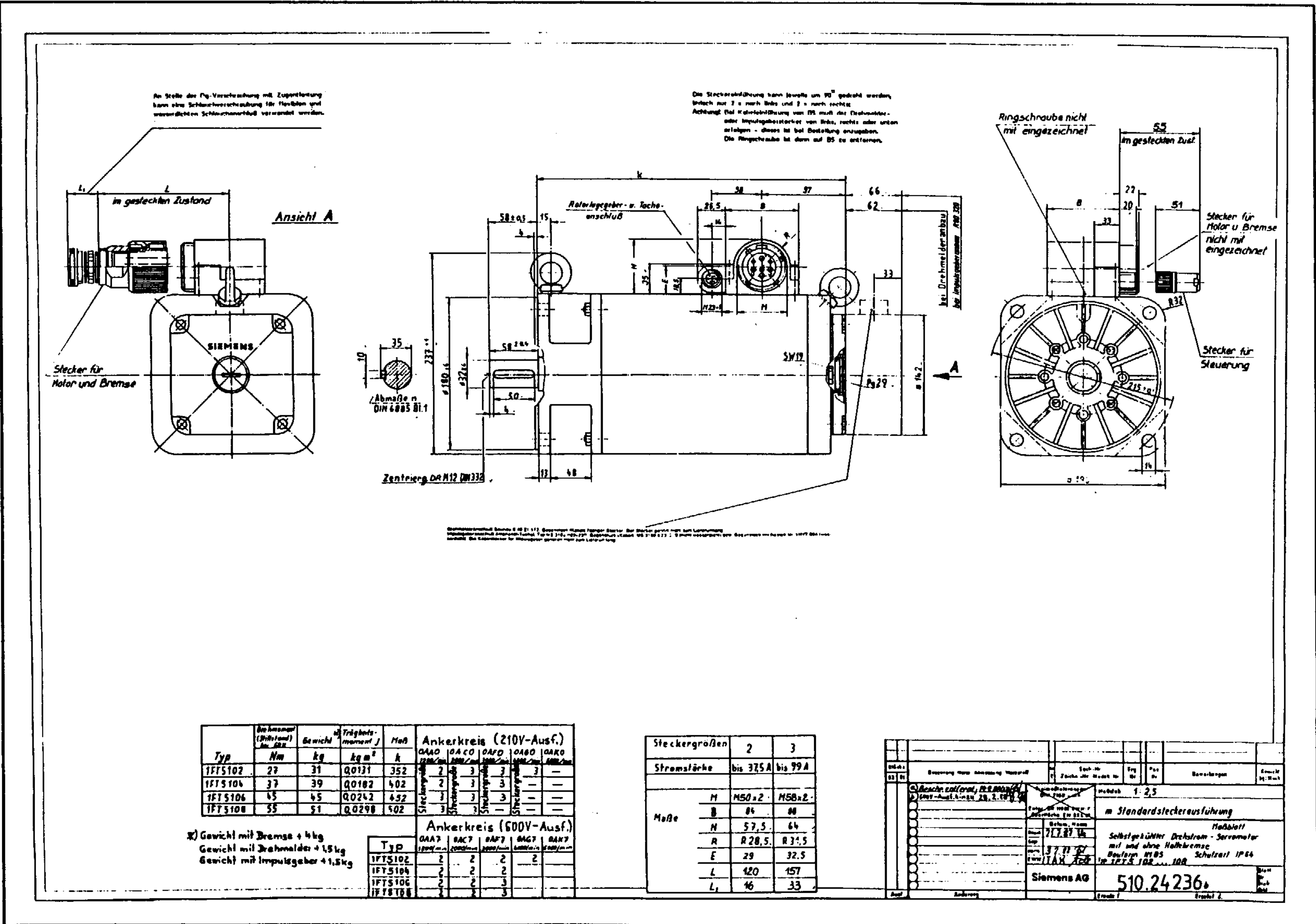
Bild 6.45 Maßblatt Drehstrom-Servomotoren IFT5102 bis IFT5108 mit Option Steckeranführung IM B5 Bitte achten Sie auf die Zuordnung der Klemmenkastengrößen für die Ankerkreise 600V. Bauform
