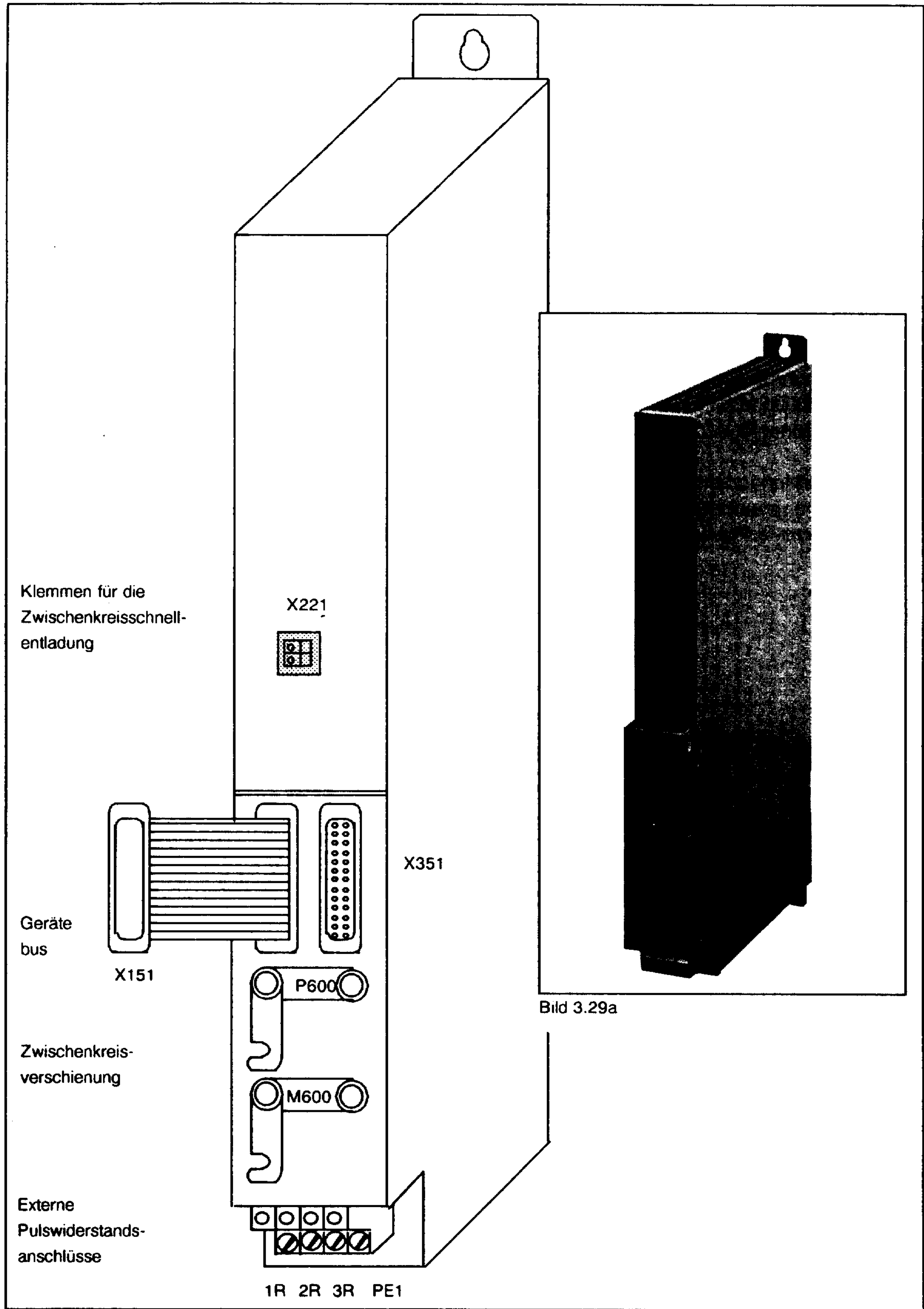
Bild 3.29 Pulswiderstandsmodul 6SC6110-0GB00
