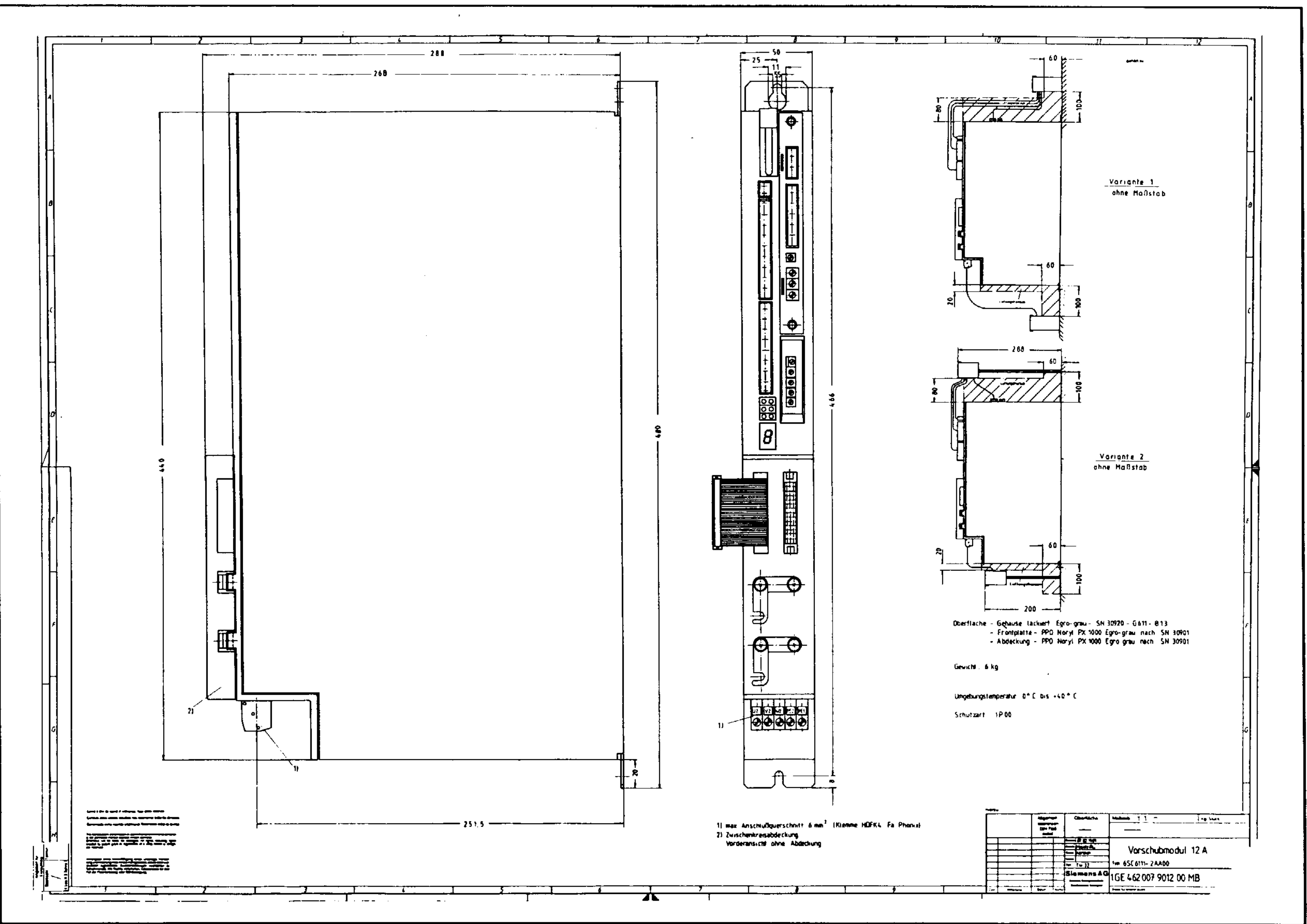
Bild 6.59 Vorschubmodul 12/24A 6SC61111-2A00
