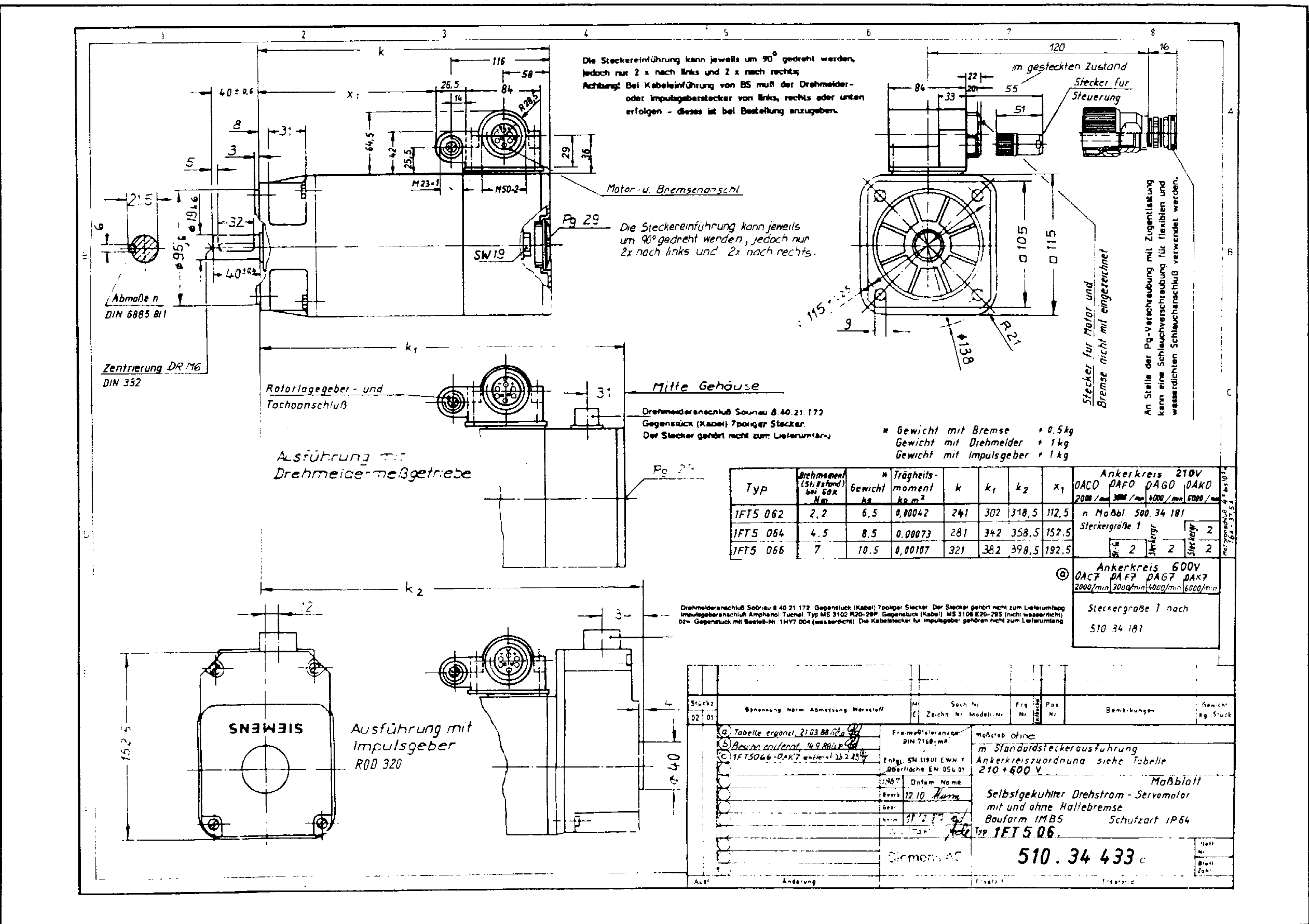
Bild 6.42 Maßblatt Drehstrom-Servomotoren 1FT5062 bis 1FT5066 mit Option Steckerausführung Bauform IM B5 Bitte achten Sie auf die Zuordnung der Klemmenkastengrößen für die Ankerkreise 600V.
