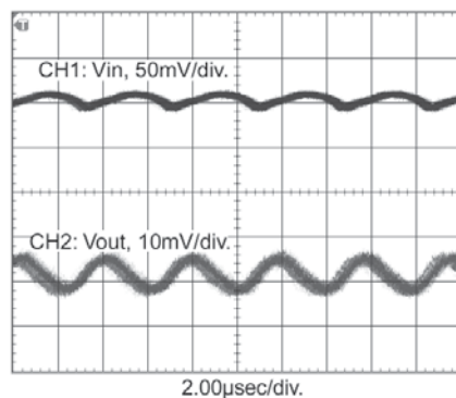
7812SR-C V_{IN} = 24\text{V} , I_{LOAD} = 40\text{mA}
