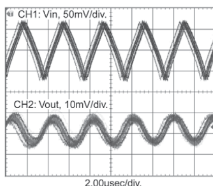
7812SR-C V_{IN} = 24\text{V} , I_{LOAD} = 400\text{mA}
