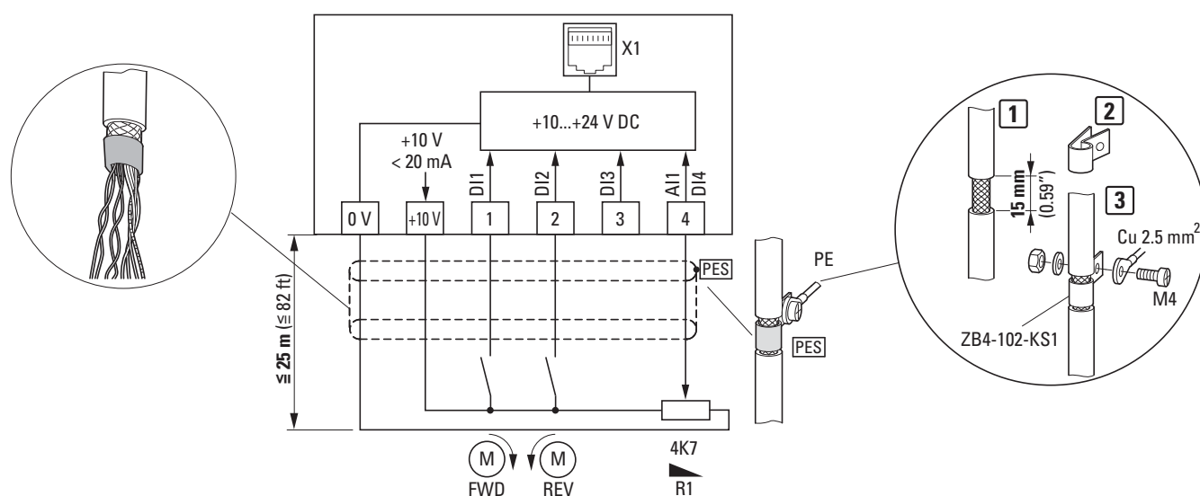
Ilustracja 41: Przykład podłączenia
