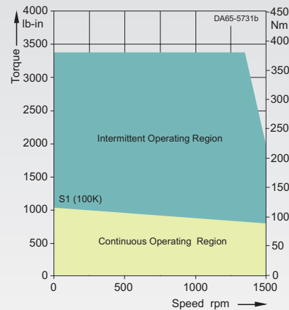
1FT6136-6AB7-....
