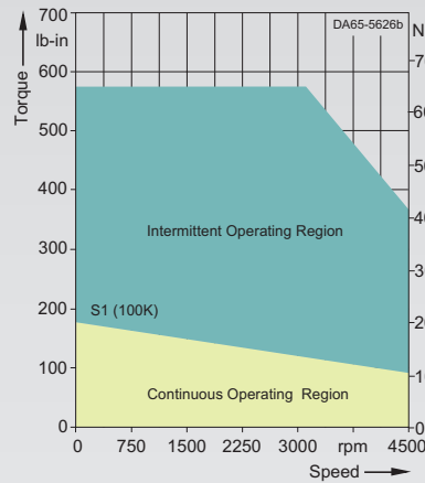
1FT6084-8AH7.-....
