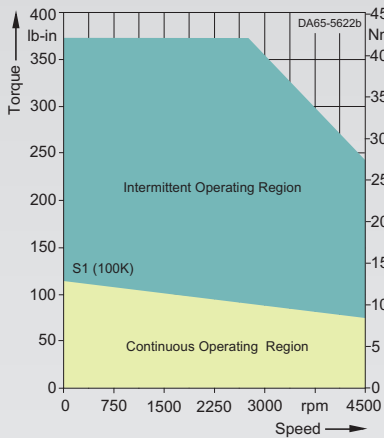
1FT6082-8AH7.-....
