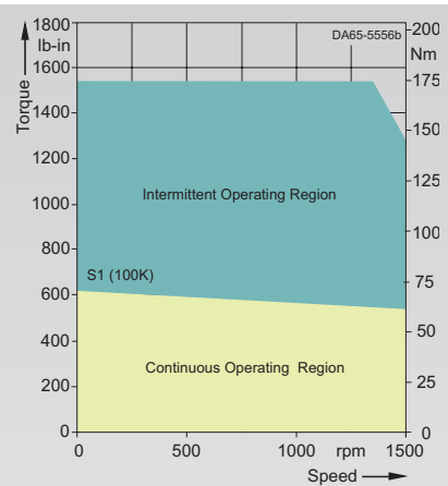
1FT6108-8AB7-....
