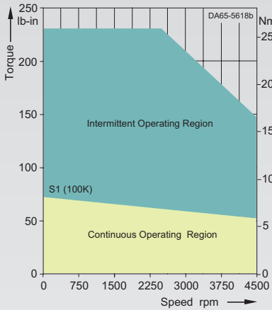
1FT6064-6AH7.-....
