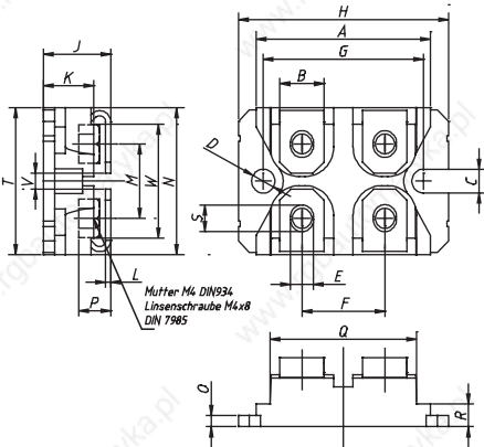
X028 ISOPLUS227™
