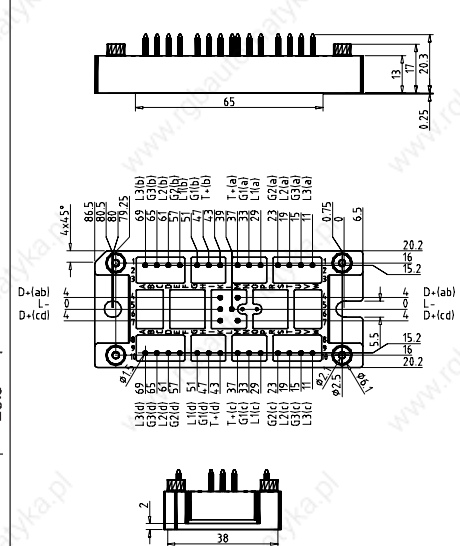
X104 V2-Pack
