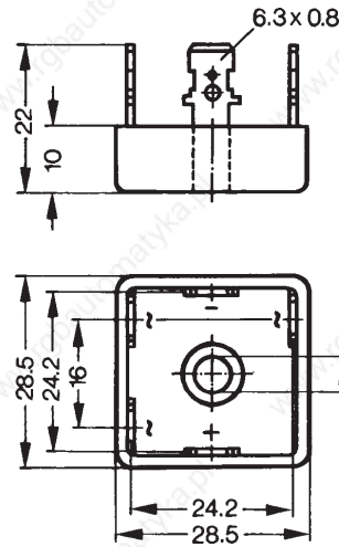
X116b FO-B-B
