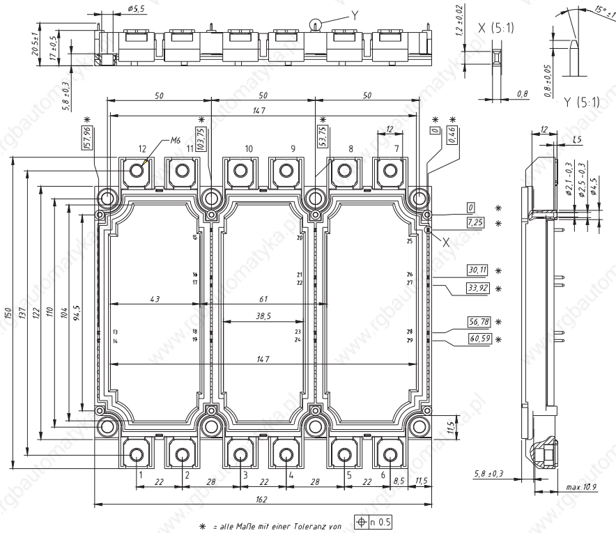
X116a FO-B-A
