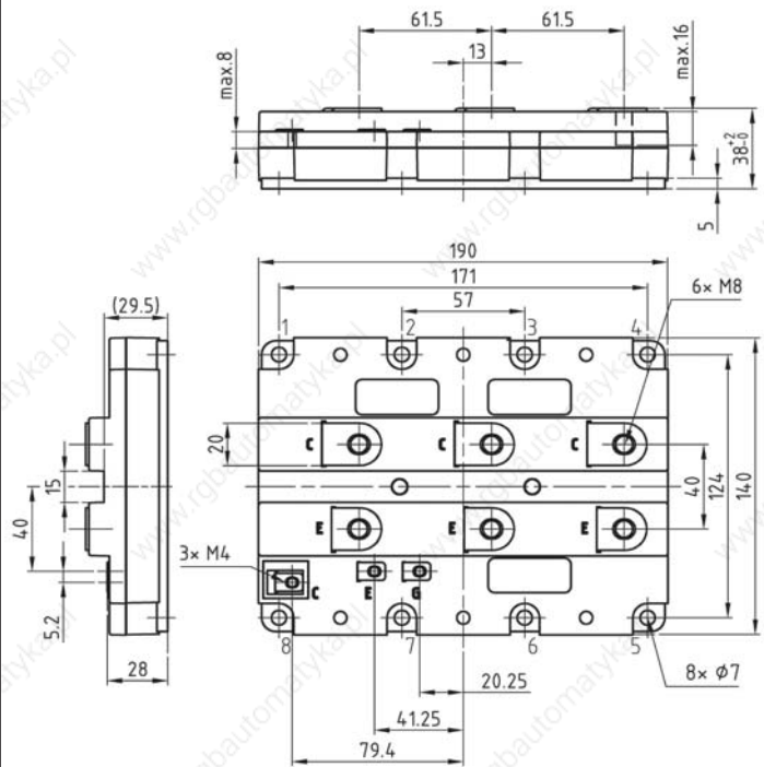
X134 E10-Pack
