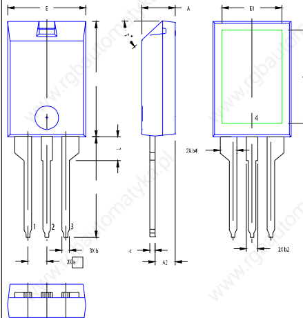
X009 PLUS220
