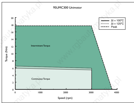
95UMC300 Unimotor
