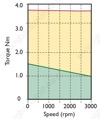
DCM 6F 30/14 Maxi Maestro DCD 200* 25/50
