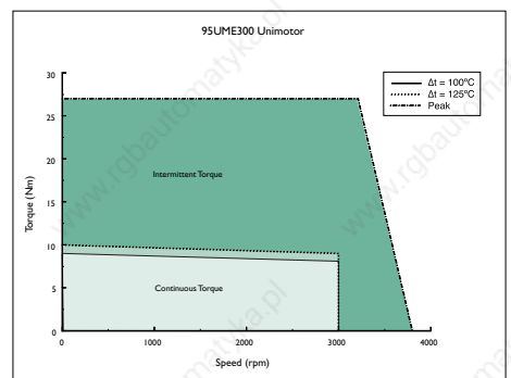
95UME300 Unimotor
