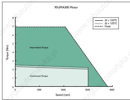
95UMA300 Unimotor
