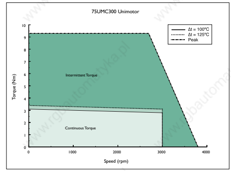
75UMC300 Unimotor
