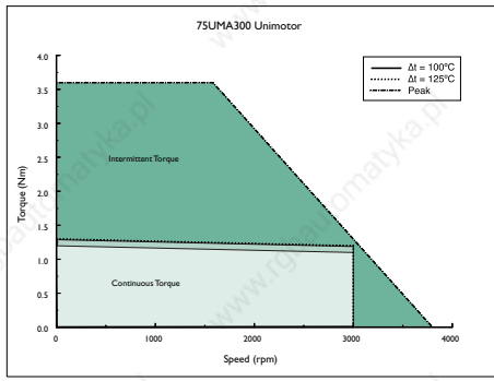
75UMA300 Unimotor
