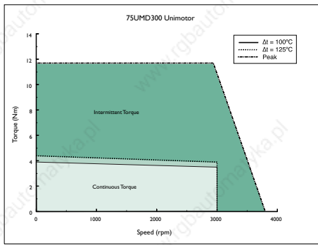
75UMD300 Unimotor
