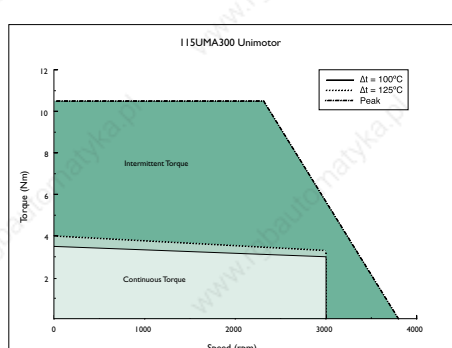
115UMA300 Unimotor
