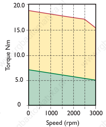
DCM 6F 30/14 Maxi Maestro DCD 200* 25/50
