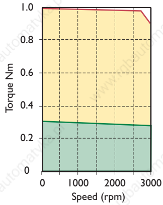
DCM 3F 30/06 Mini Maestro DCD 60* 12/28
