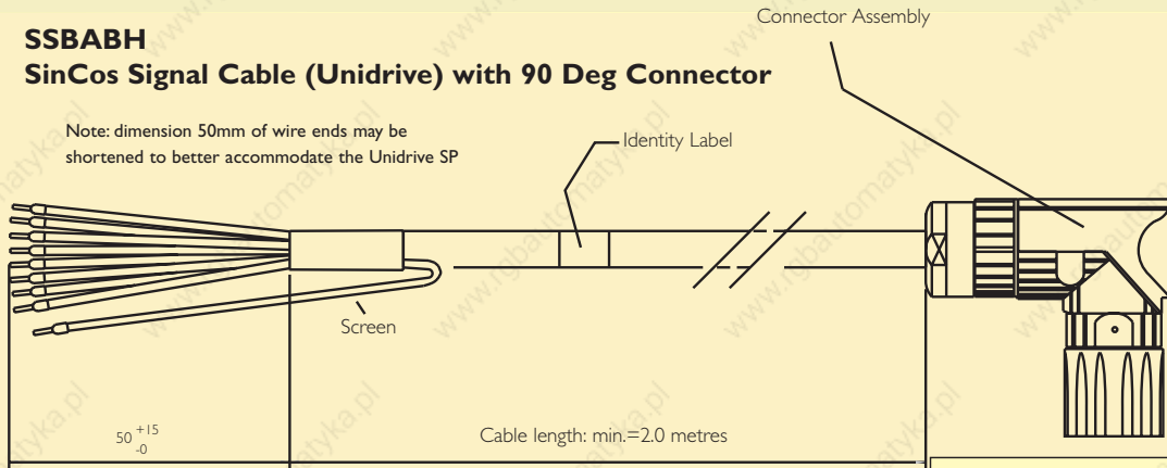
INTERCONNECTRON 12 WAY
