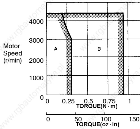
• SGM-01A (V)
