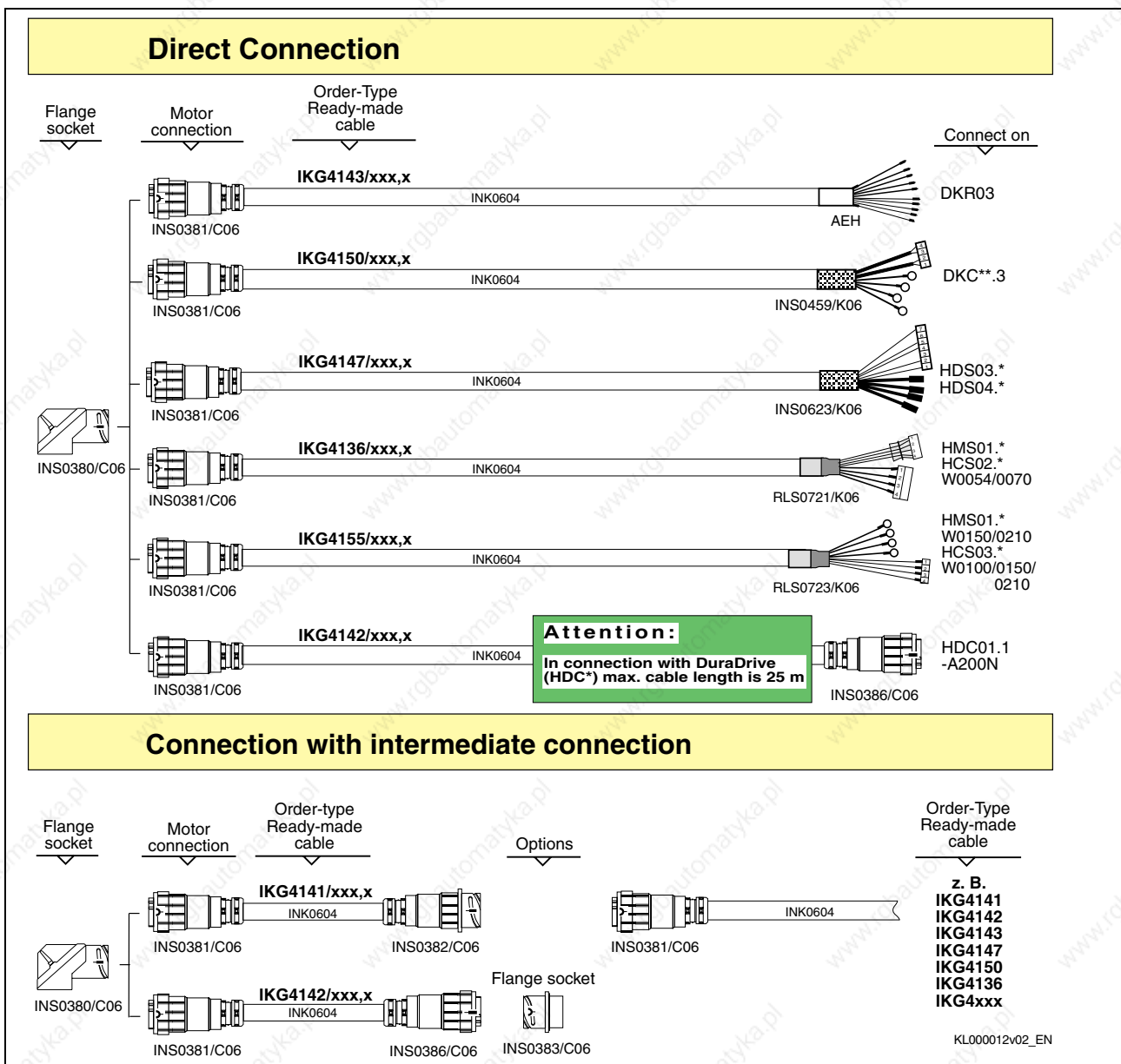
Fig. 17-9: Kabelausswahl INS0380 – 6,0mm 2
