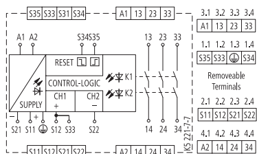
ESR4-NO-30...(AC 115/230 V)
