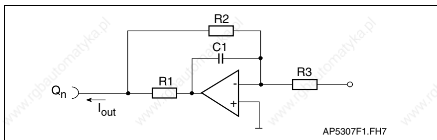
Fig. 6-26: Output load
