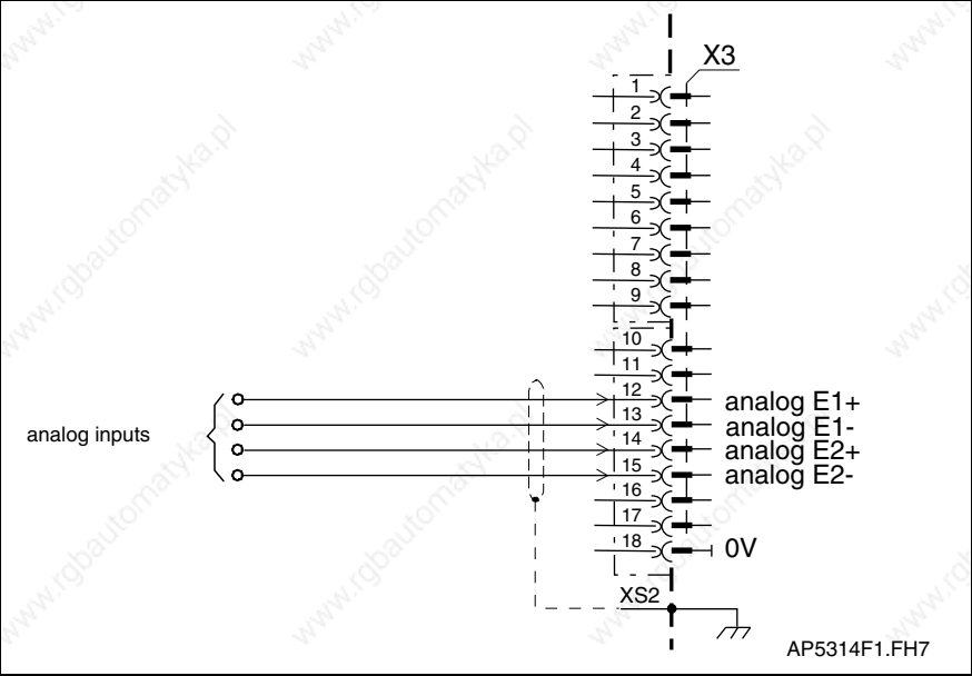
Fig. 4-76: Analog inputs
