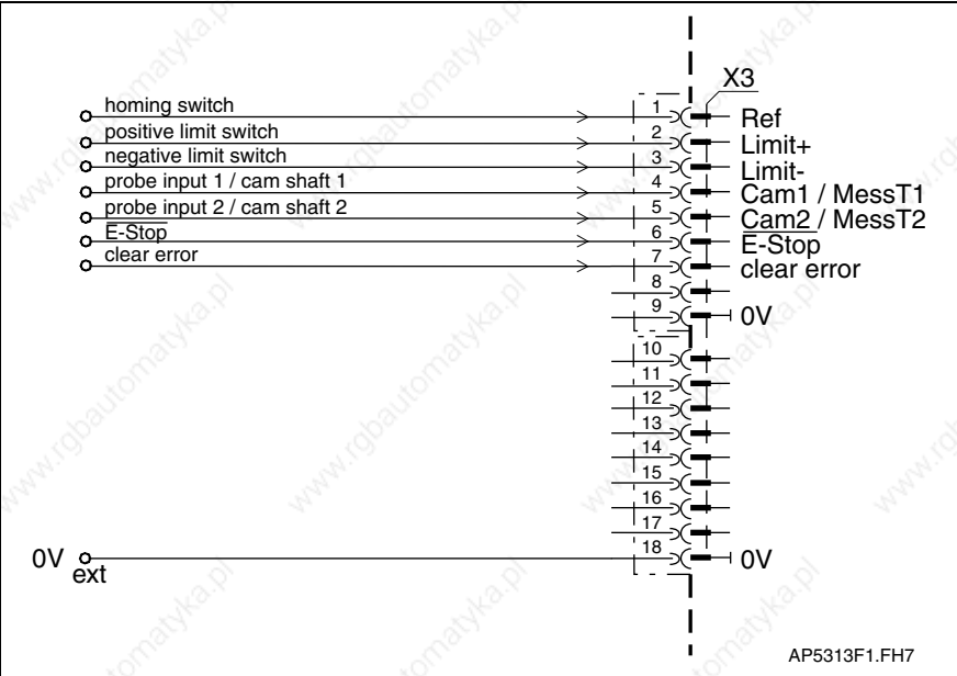
Fig. 4-66: Digital inputs
