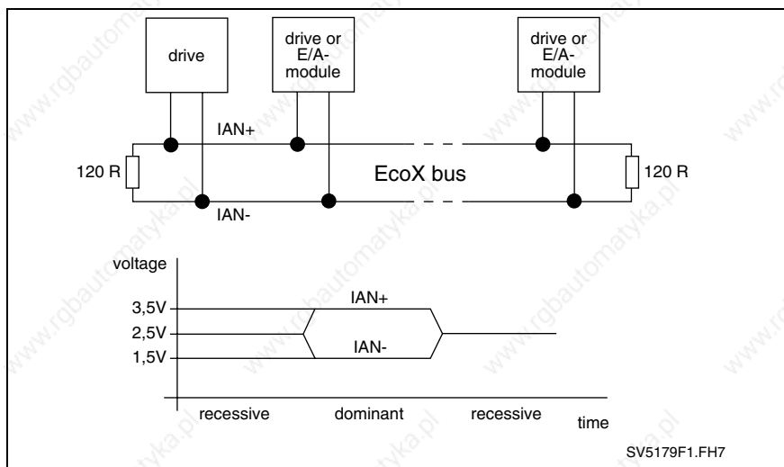
Fig. 4-137: EcoX interface
