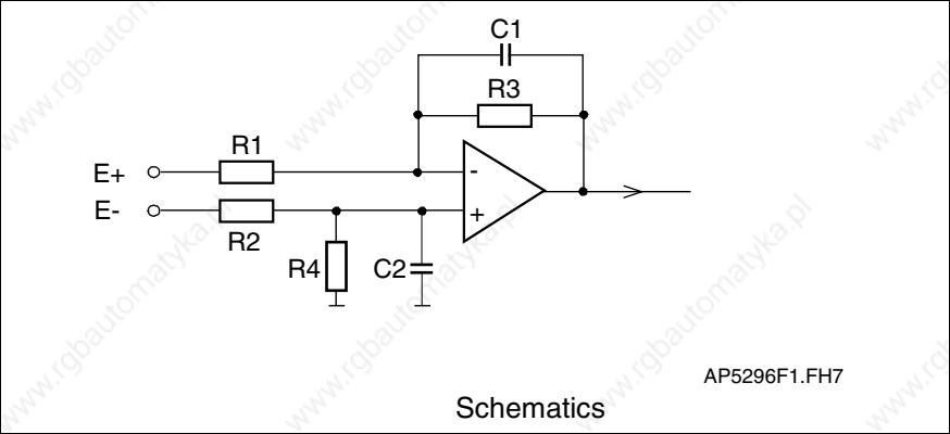
Fig. 4-76: Analog inputs
