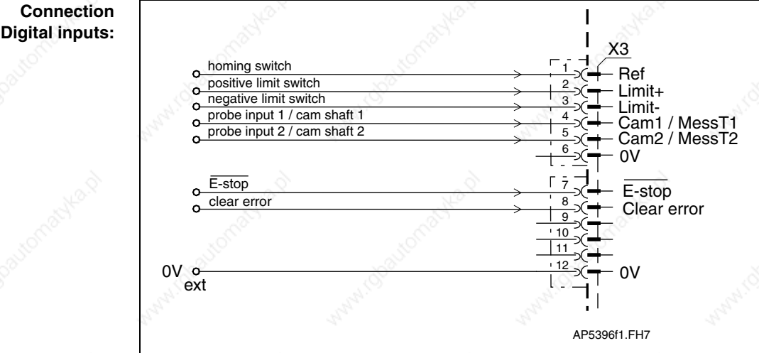
Fig. 5-38: Digital inputs
