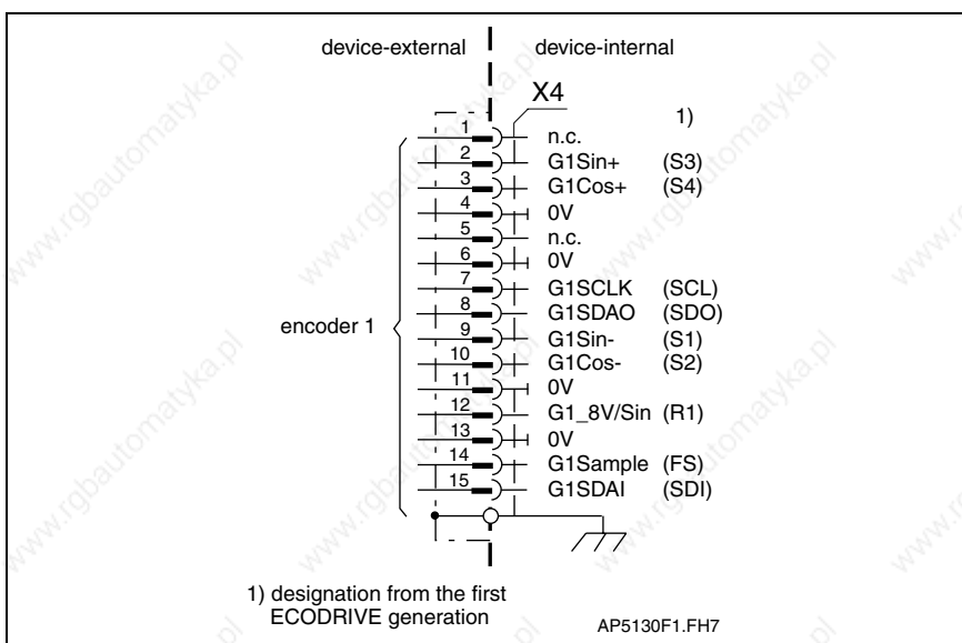
Fig. 4-84: Encoder 1
