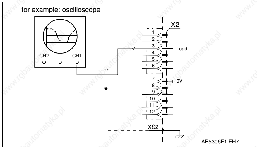
Fig. 6-26: Output load
