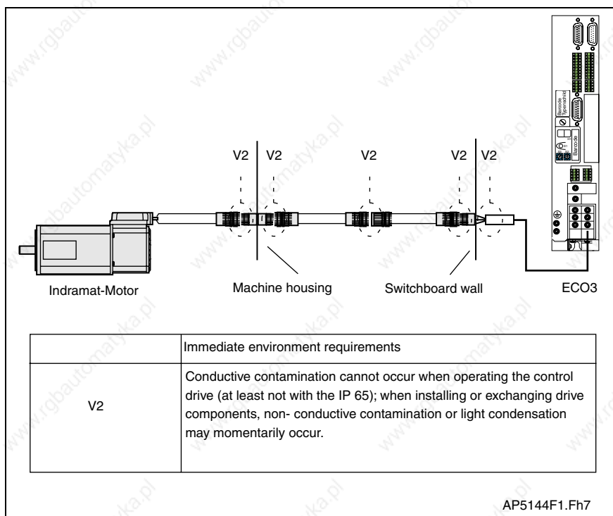
Fig. 15-2: Dirt contamination per DIN VDE 0160
