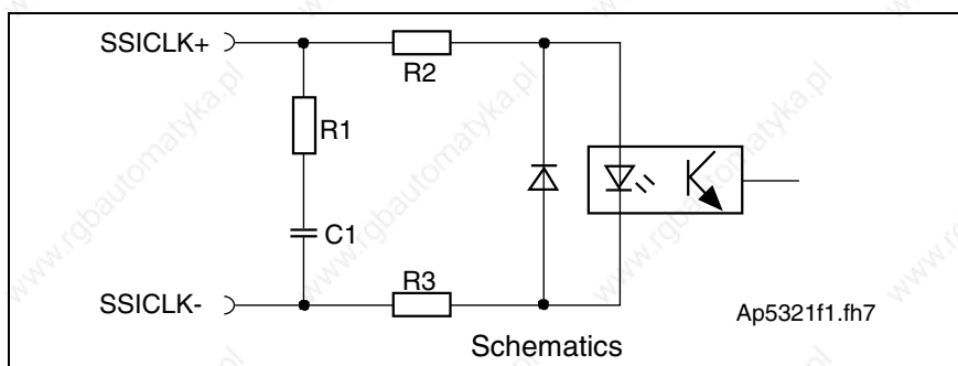
Fig. 4-129: Output of absolute actual position value in SSI format
