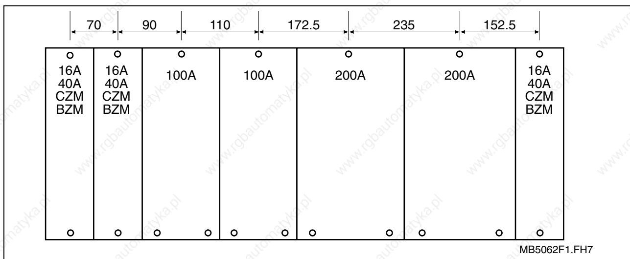
Fig. 12-16: Module widths
