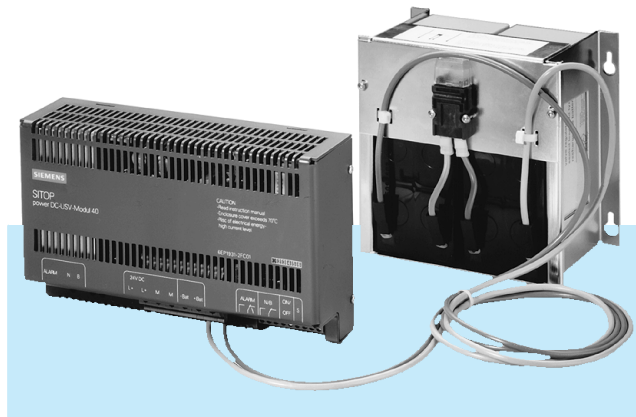
Bild 3/9 Unterbrechungsfreie Stromversorgung special line 24 V/40 A und Batteriemodul 24 V/7 Ah
