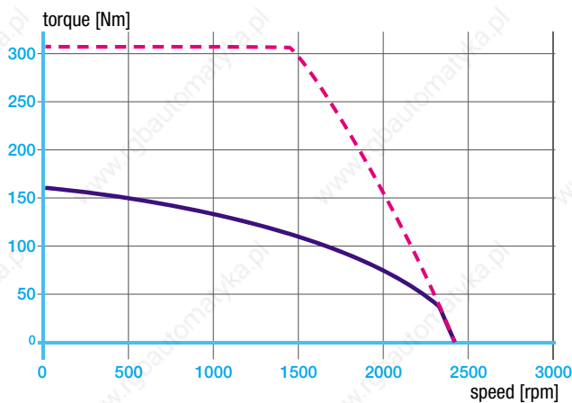
DT10-145-20-xxW-2000-B5
