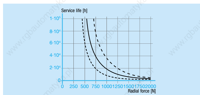
DT7-72-20-xxW-5000-B5
