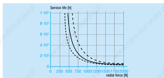
DT7-11-20-xxO-3500-B5 · DT7-17-20-xxO-3500-B5
