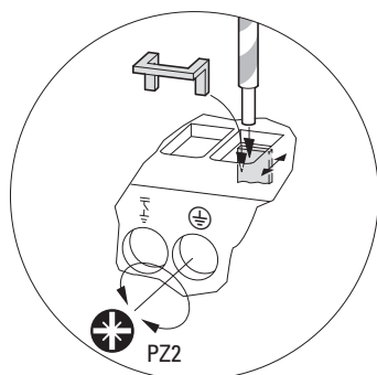
Ilustracja 32: Przewód PE wetknięty za zworką EMC (zacisk od tyłu do przodu)
