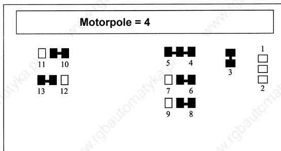
Layout der Jumper auf der Kunden - Steckplatine Die Zahlen entsprechen Brücke P1 - P13
