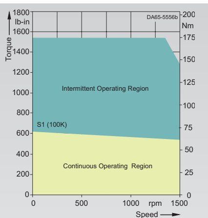
1FT6108-8AB7-....
