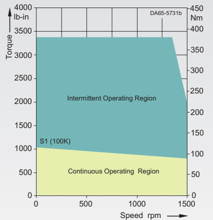
1FT6136-6AB7-....
