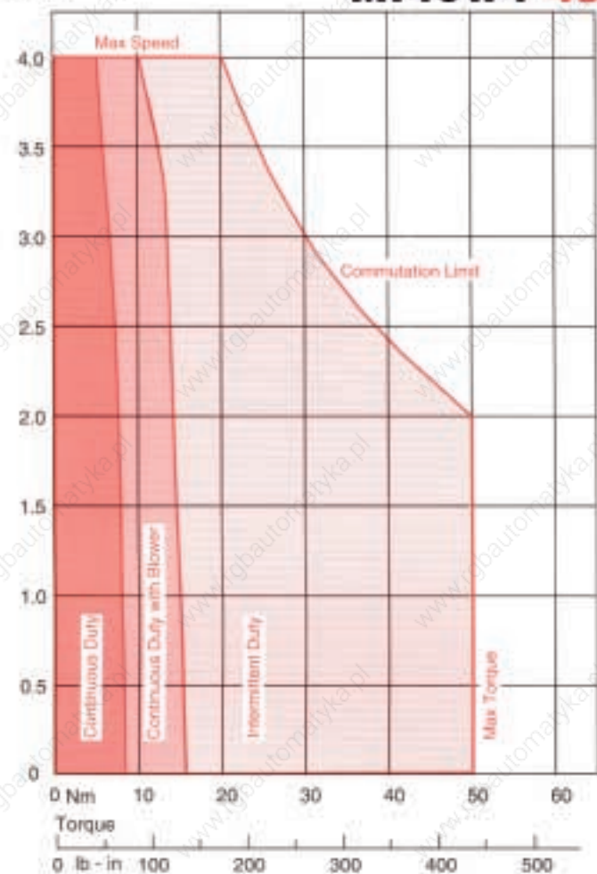
Speed Kr.p.m. MT40W4-45
