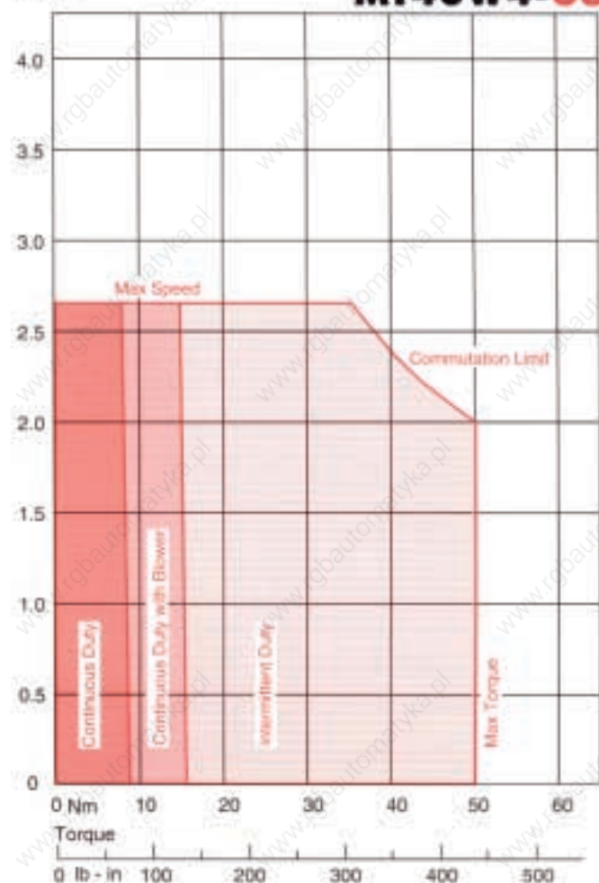
Speed Kr.p.m. MT40W4-68
