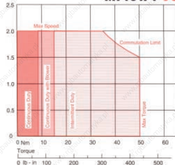
Speed Kr.p.m. MT40W4-90
