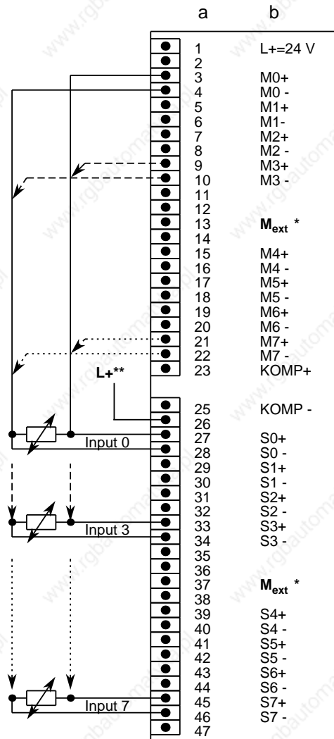
6ES5 465-7LA13
