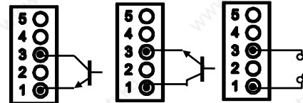
Fig.61.2. Ejemplos de conexión. PNP, NPN o contacto libre.
