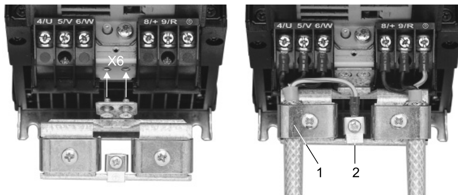
[1] Zacisk ekranujący
