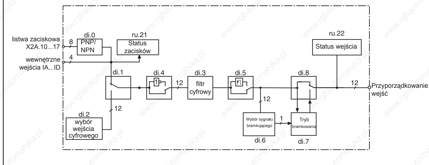
Ryc. 6.3.2.a Cyfrowe wejścia w układzie sterowania PNP (di.0 = 0)
