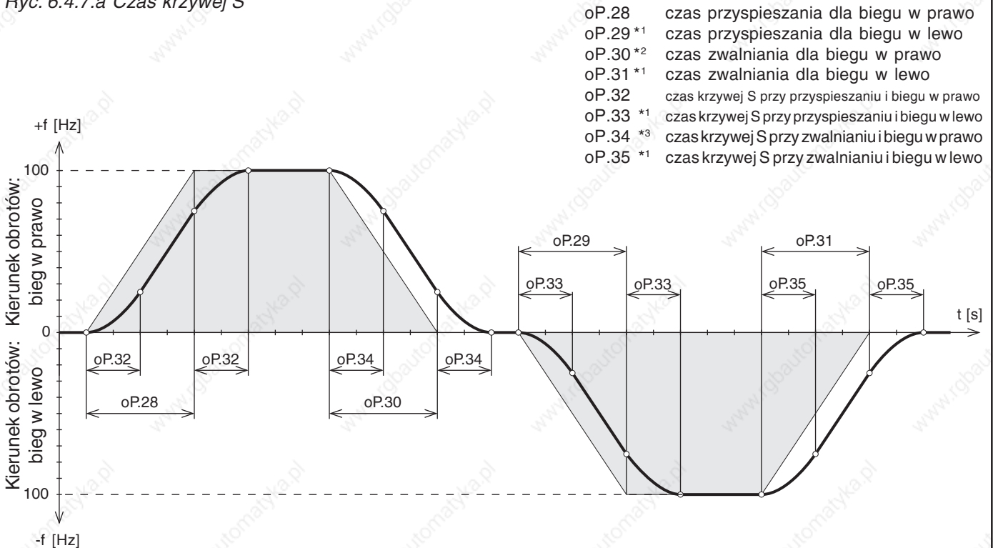
Ryc. 6.4.7.a Czas krzywej S
