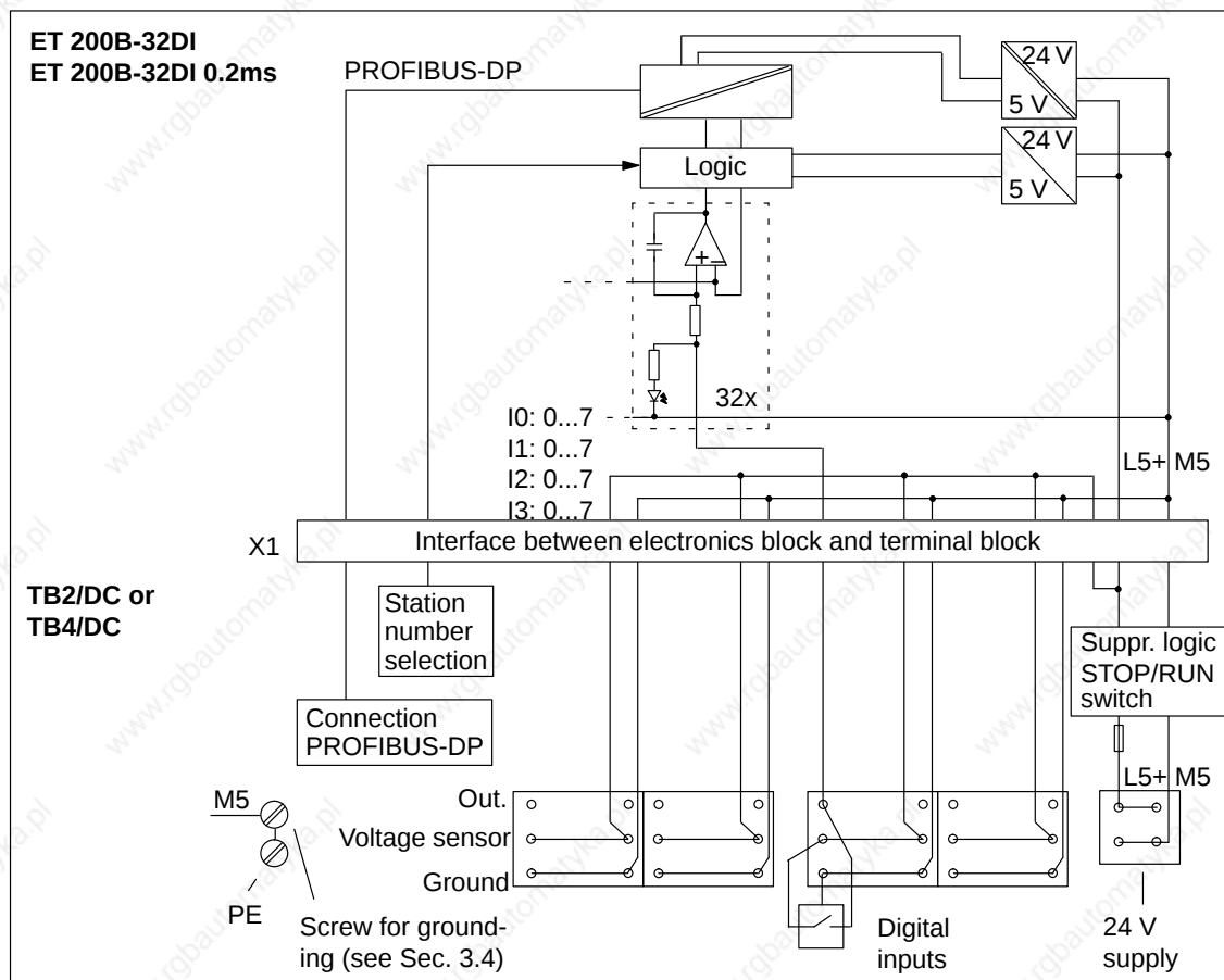
Figure 7-24 Block Diagram: ET 200B-32DI (6ES7 131-0BL00-0XB0) or ET 200B-32DI 0.2ms (6ES7 131-0BL10-0XB0) and TB2/DC or TB4/DC
