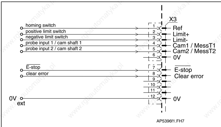
Fig. 5-38: Digital inputs
