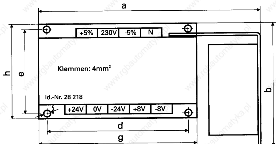
Abb. 8 Encoderversorgung 230V
