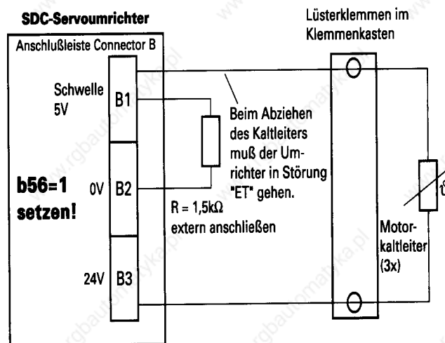
Abb. 5 Kaltleiteranschluß im Klemmenkasten
