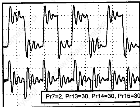
Abb. 13 Beispiel zur optimalen Reglereinstellung
