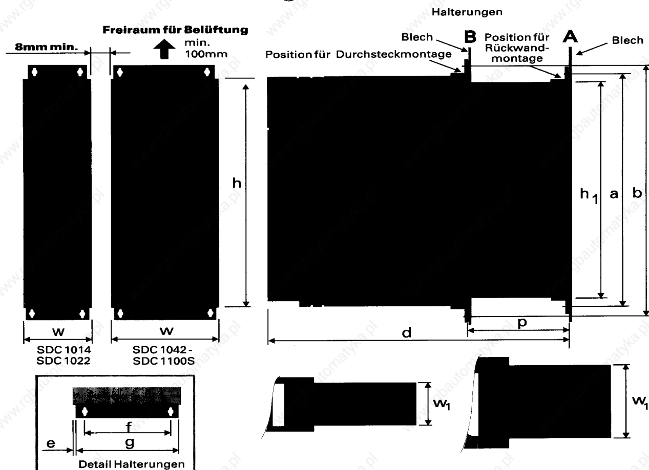
Abb. 1 Abmessungen
