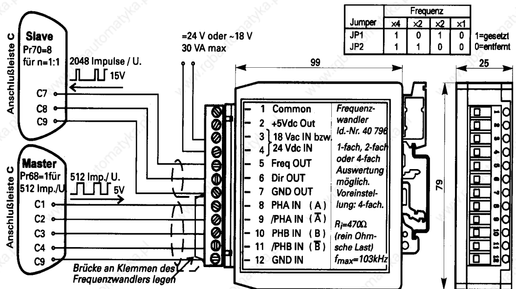
Abb. 15 Anschlußbild für Synchronregelung mit Frequenzumsetzer
