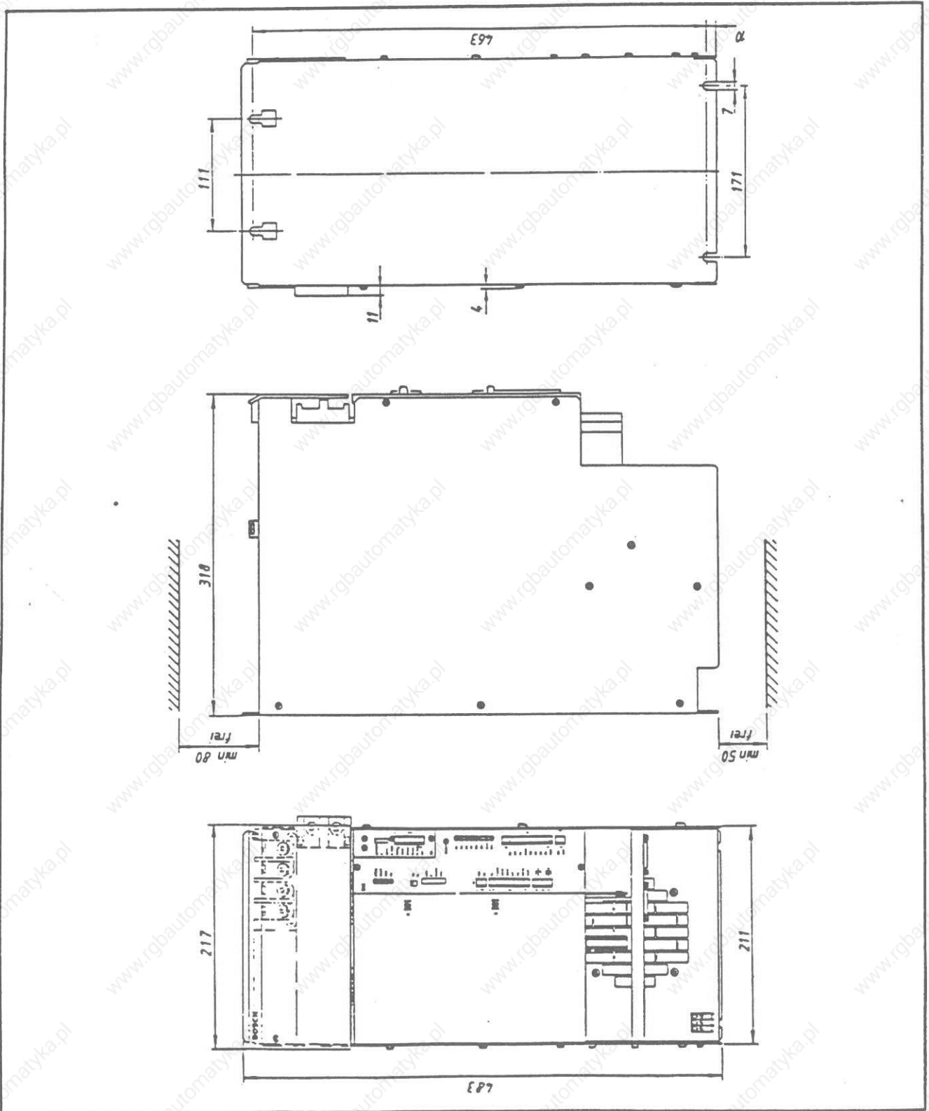
Maßbild SM 75/150
