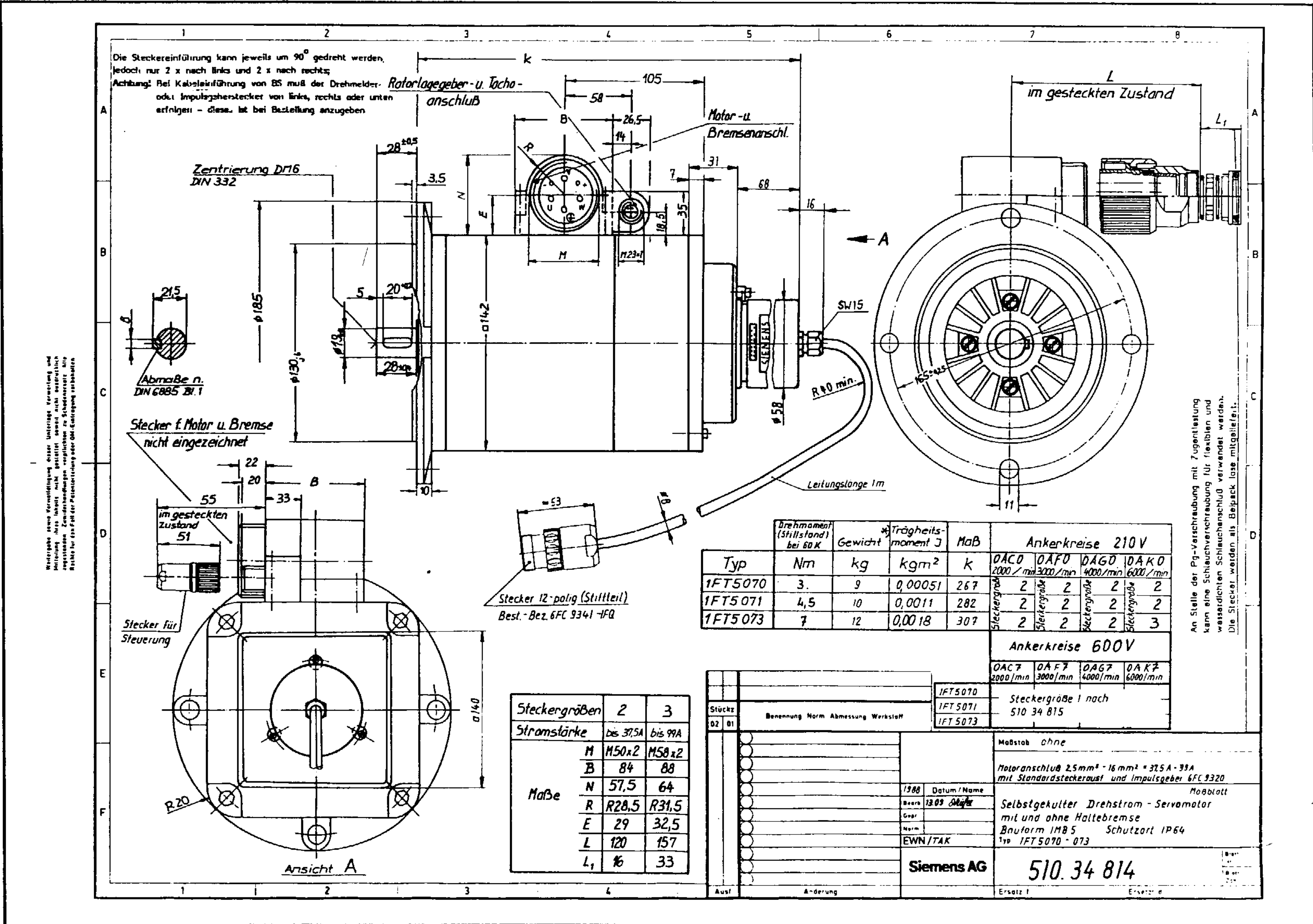
Bild 6.51 Maßblatt Drehstrom-Servomotoren 1FT5070, 1FT5071 und 1FT5073 mit Option Steckerausführung Bauform IM B5 Bitte achten Sie auf die Zuordnung der Klemmenkastengrößen für die Ankerkreise 600V.
