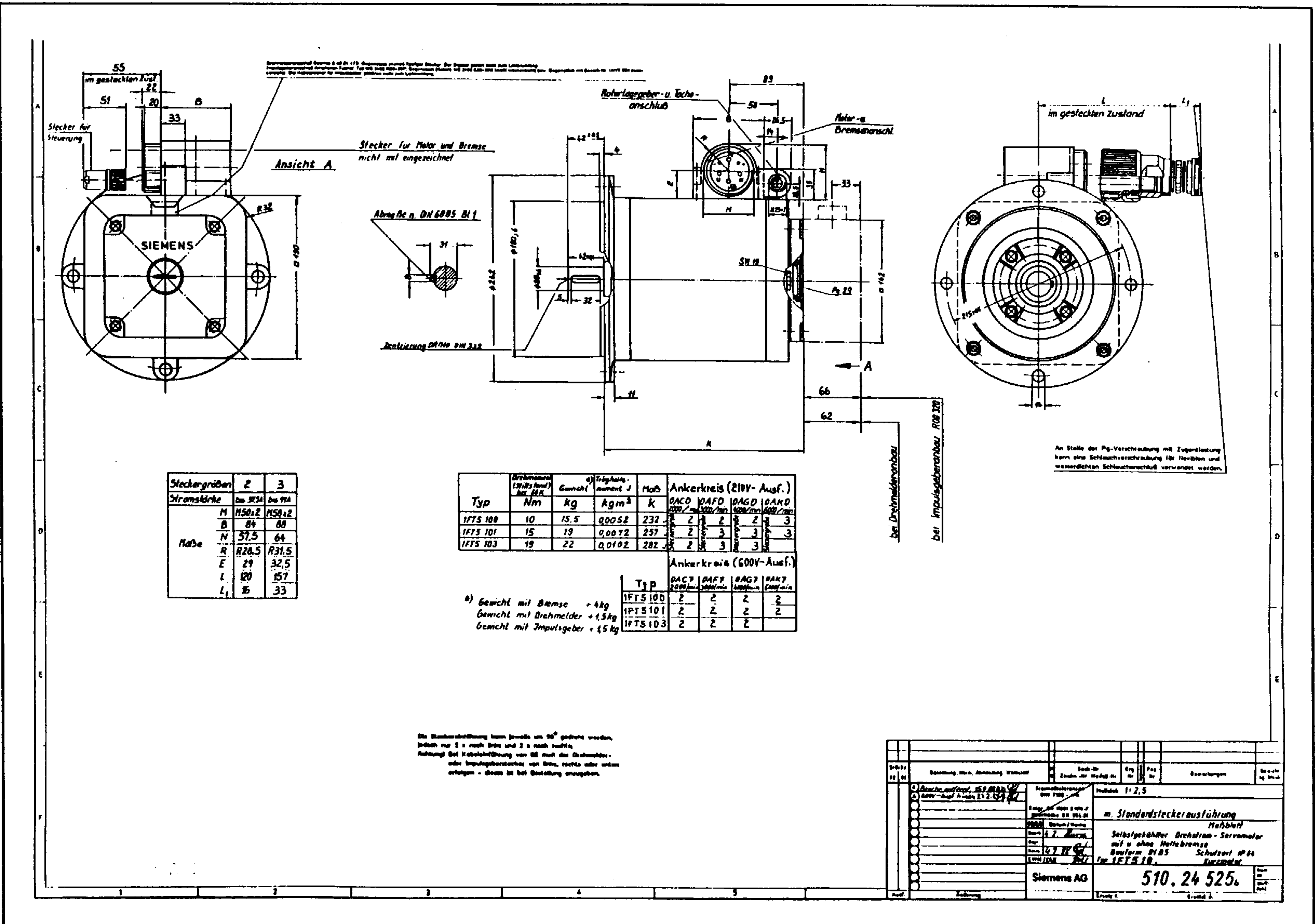
Bild 6.53 Maßblatt Drehstrom-Servomotoren 1FT5100, 1FT5101 und 1FT5073 mit Option Steckerausführung Bauforn IM B5 Bitte achten Sie auf die Zuordnung der Klemmenkastengrößen für die Ankerkreise 600V.
