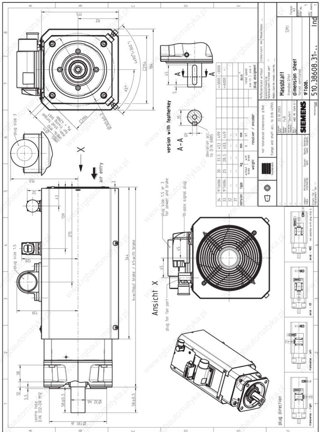
Figure 5-9 1FT608□-□S□DQ
