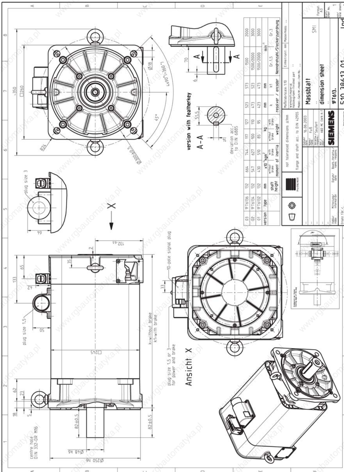
Figure 5-7 1FT613□-□A□plug□DQ
