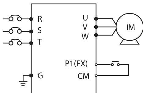
[Schemat połączeń]
