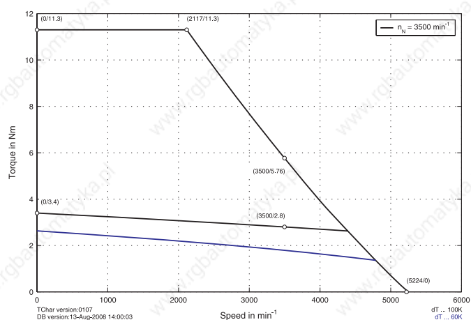
ACOPOS
