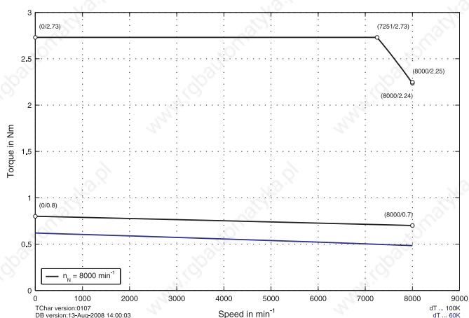
ACOPOS
