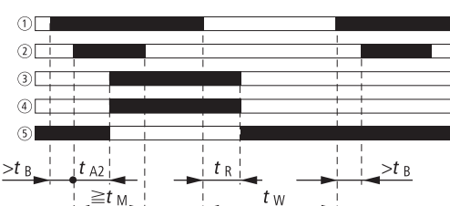
Uruchomienie ręczne z kontrolą przycisku reset
