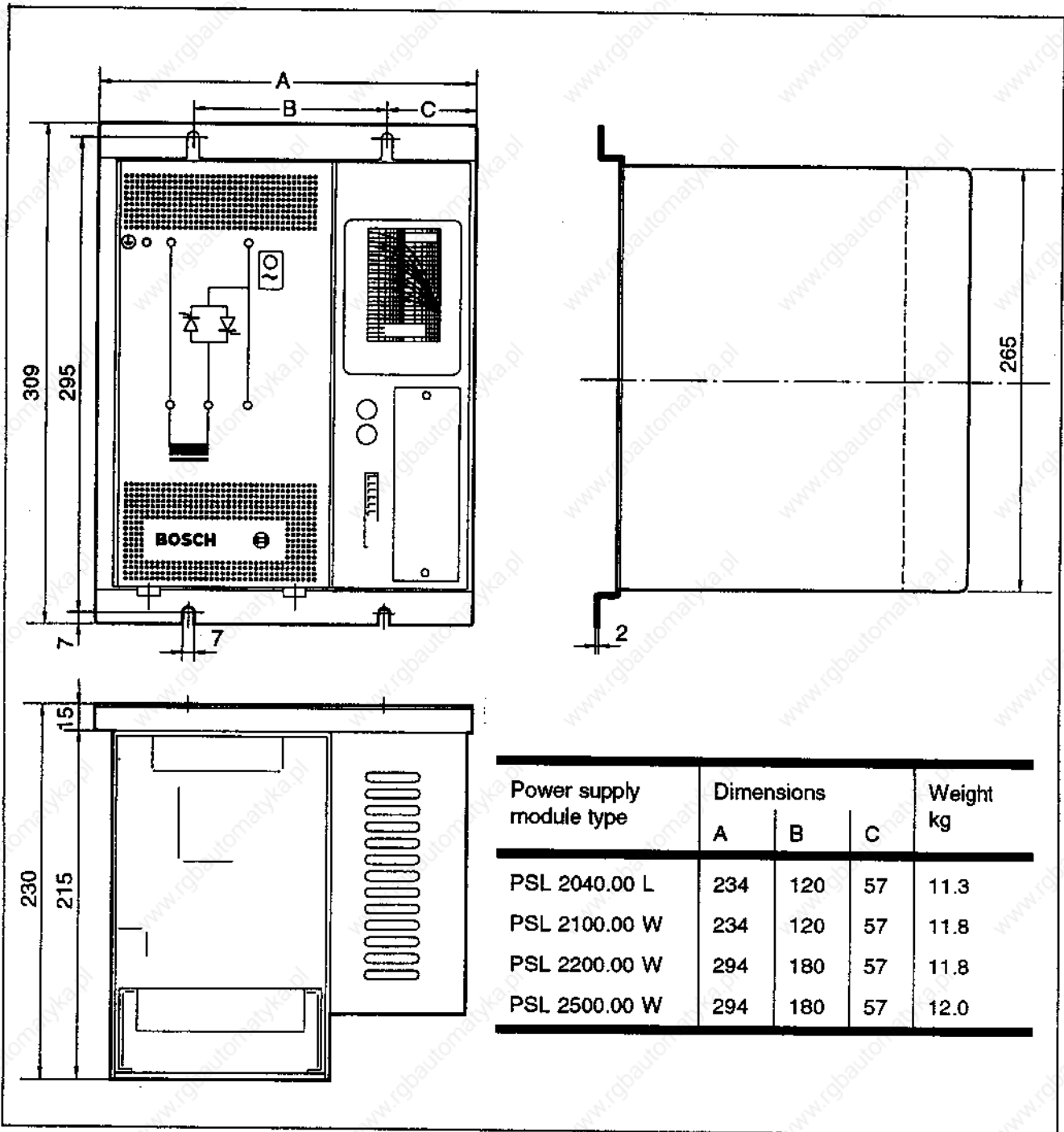
Fig. 2.6 Dimensions
