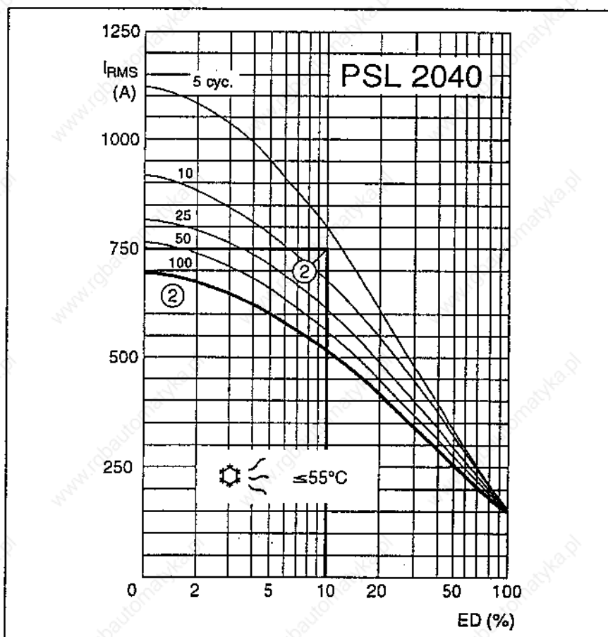
Fig. 7.3 Load diagram
