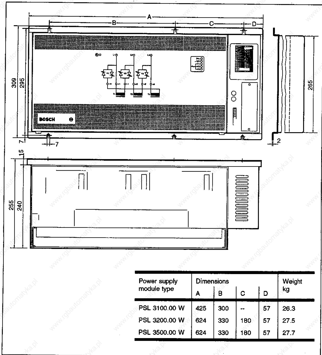
Fig. 3.5 Dimensions
