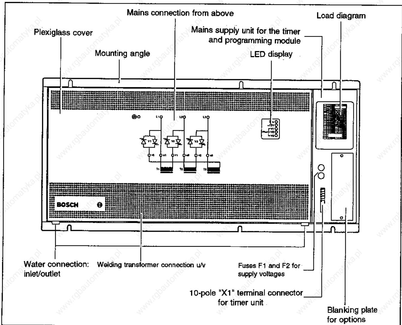
Fig. 3.1 PSL 3000
