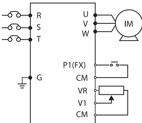
[Schemat połączeń]
