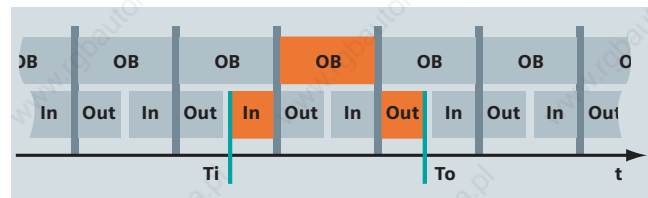
Tryb izochroniczny i synchroniczny przetwarzania sygnału
