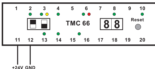
Fig. 5.1-1: Supply wiring
