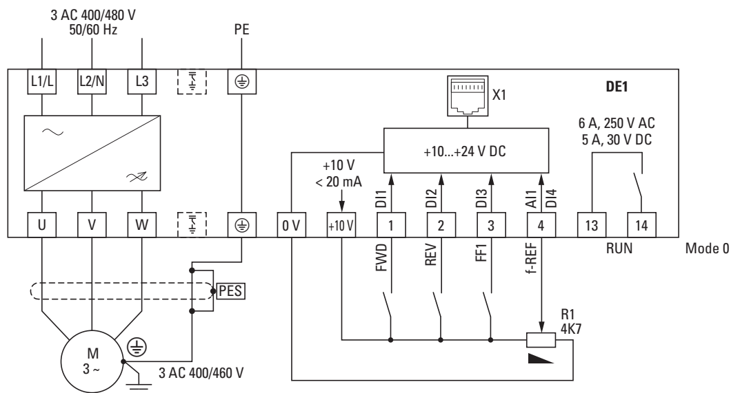
Ilustracja 51: Schemat blokowy DE1-34...NN-... Rozrusznik silnikowy z regulacją prędkości z trójfazowym napięciem zasilającym i bez wewnętrznego filtra przeciwzakłóceńowego
