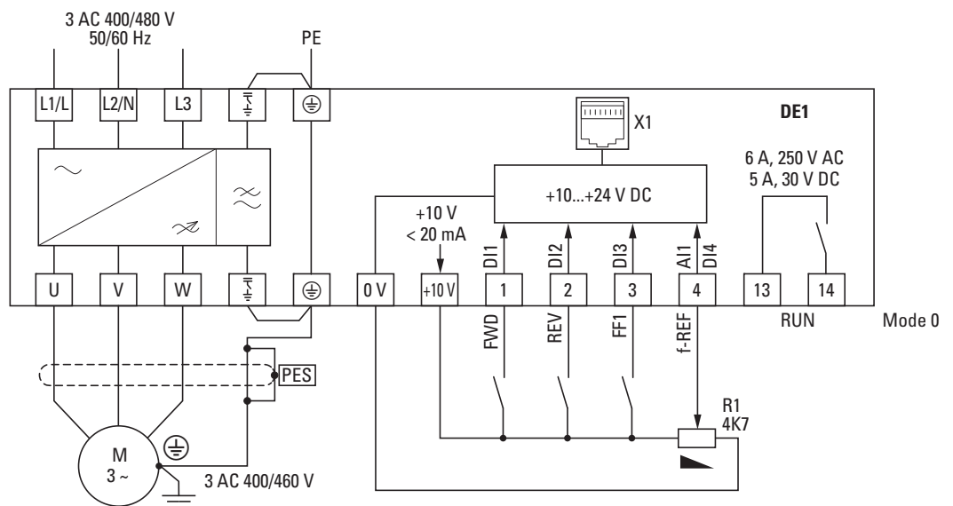
Ilustracja 50: Schemat blokowy DE1-34...FN-... Rozrusznik silnikowy z regulacją prędkości z trójfazowym napięciem zasilającym i wewnętrznym filtrem przeciwzakłóceńowym
