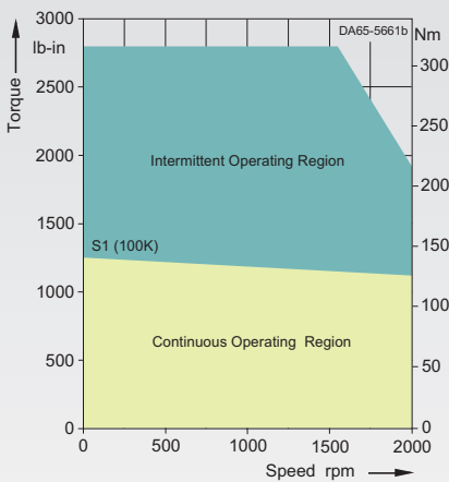
1FT6134-6SC7.-....
