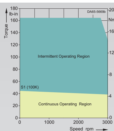
1FT6044-4AF7-....
