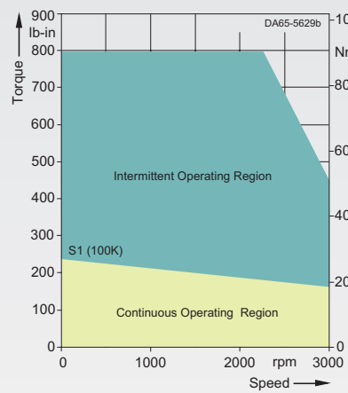
1FT6086-8AF7-....
