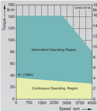
1FT6061-6AH7.-....
