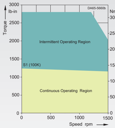
1FT6134-6SB7-....
