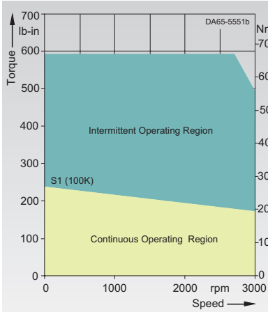
1FT6102-8AF7.-....
