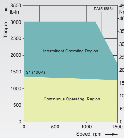
1FT6136-6SB7-....
