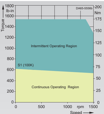
1FT6108-8AB7-....
