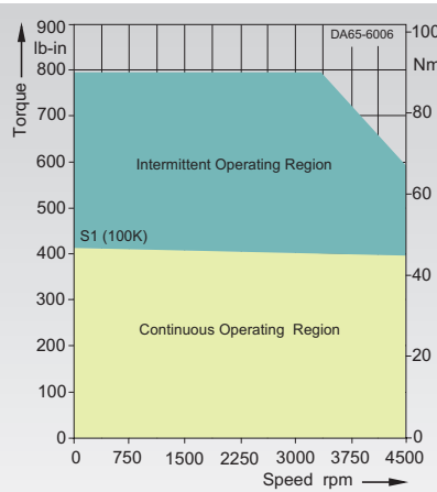
1FT6086-8WH7.-....
