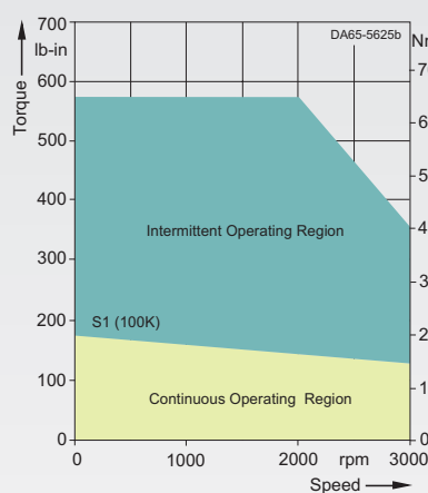
1FT6084-8AF7-....
