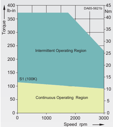
1FT6082-8AF7-....
