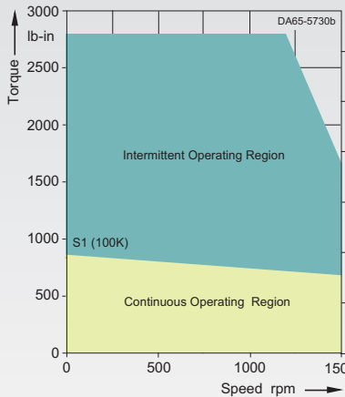
1FT6134-6AB7-....
