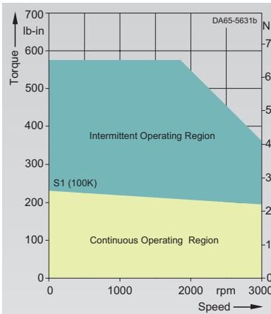
1FT6084-8SF7.-....
