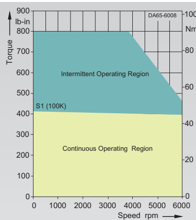
1FT6086-8WK7.-....
