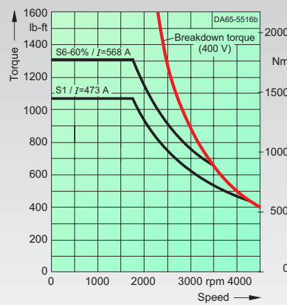
1PL6228-4.F. 1) max. breakdown torque: 2630 lb-ft/3566 Nm
