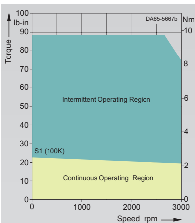
1FT6041-4AF7-....
