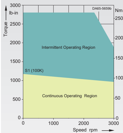
1FT6132-6SF7.-....
