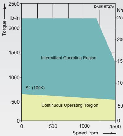
1FT6132-6AB7-....
