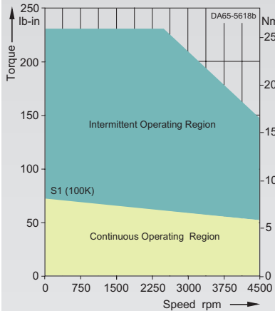
1FT6064-6AH7.-....
