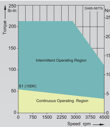
1FT6062-6AH7.-....
