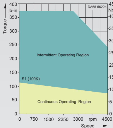
1FT6082-8AH7.-....
