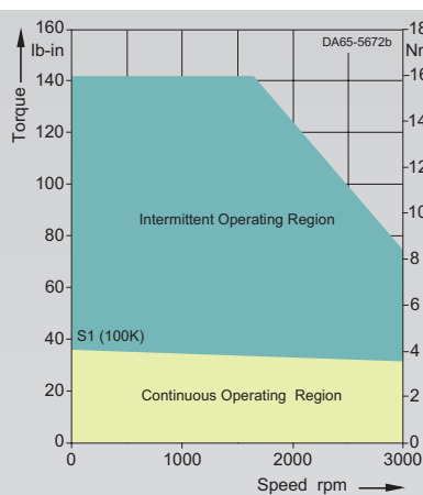
1FT6061-6AF7-....
