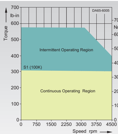
1FT6084-8WH7.-....
