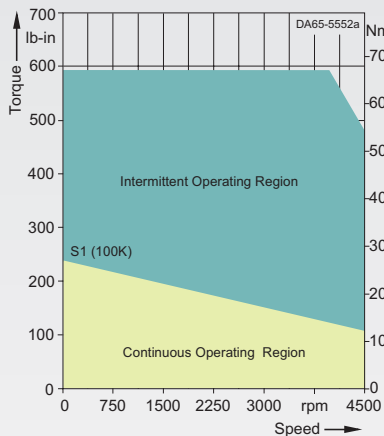
1FT6102-8AH7.-....
