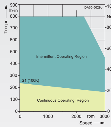
1FT6086-8AF7-....
