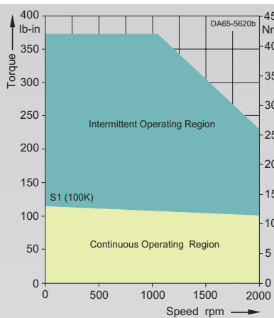
1FT6082-8AC7-....
