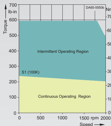
1FT6102-8AC7-....
