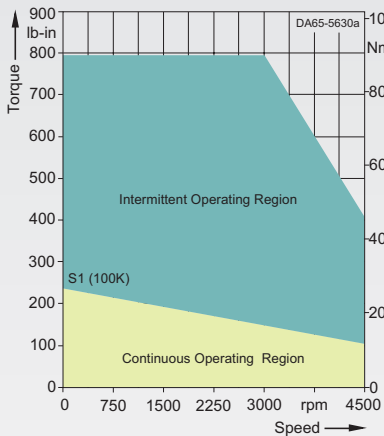
1FT6086-8AH7.-....
