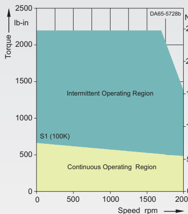
1FT6132-6AC7-....
