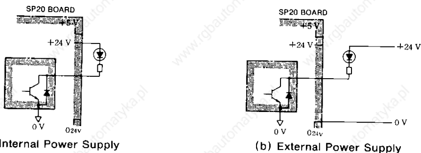
Fig 17 5 Input Circuits
