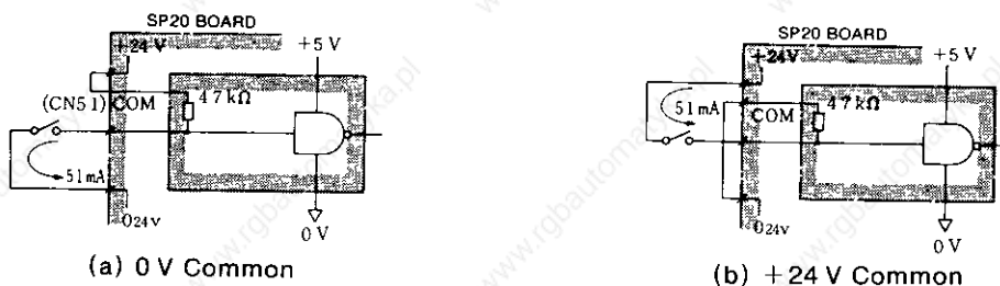
Fig 17 5 Input Circuits
