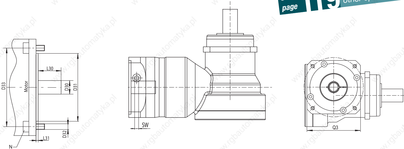
OP 2: Motoranbaumöglichkeiten
