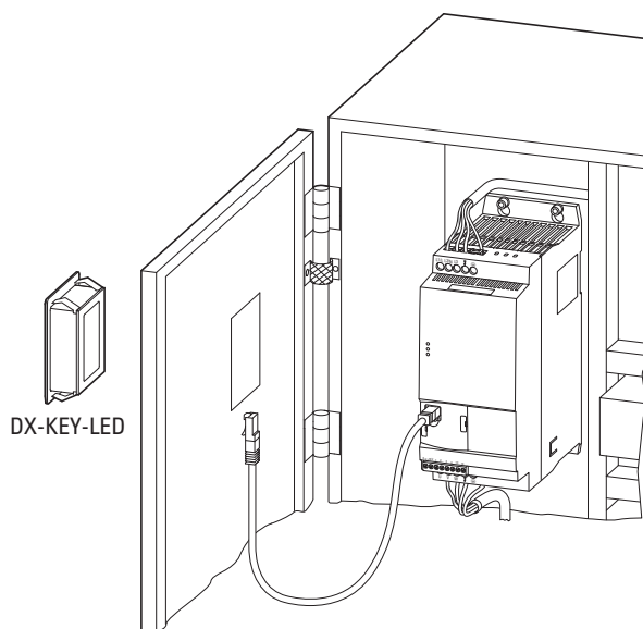
Ilustracja 79: Montaż w drzwiach szafy sterowniczej
