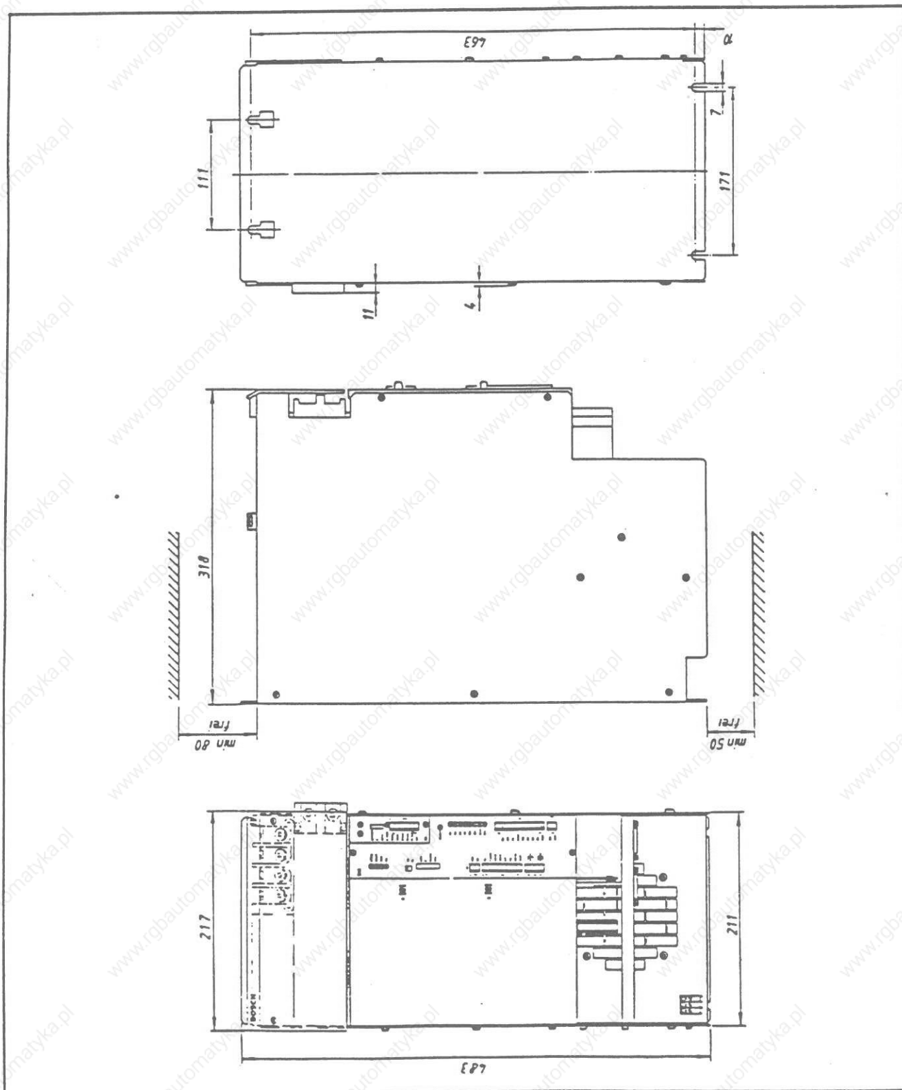
Maßbild SM 75/150
