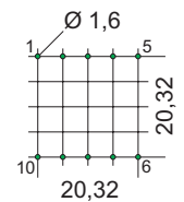
Ansicht auf Stiftseite Raster = 5,08 mm
