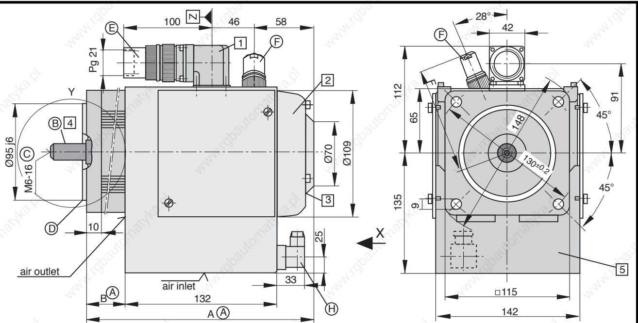
Detail Y
